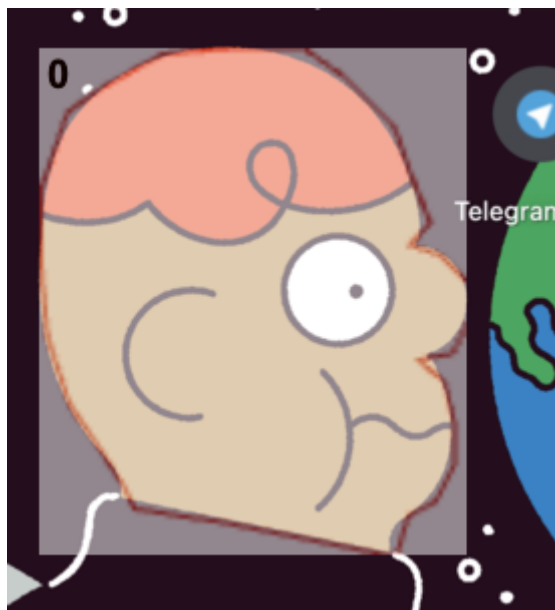
Рисунок 1 - Область многоугольник
