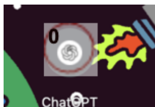
Рисунок 3 - Область окружности
