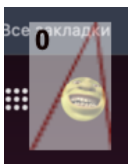
Рисунок 5 - Область треугольник
