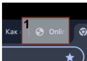
Рисунок 4 - Область прямоугольника
