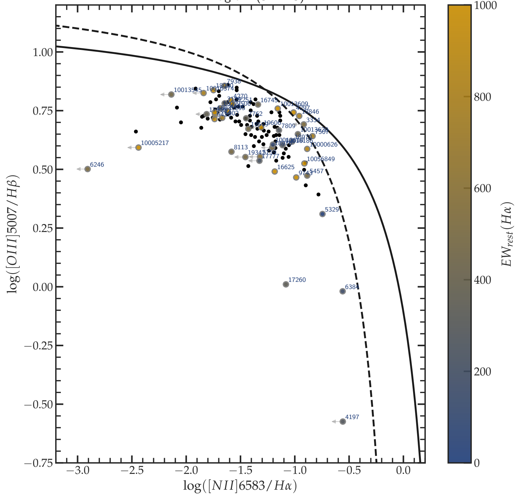
BPT Diagram (JADES)
