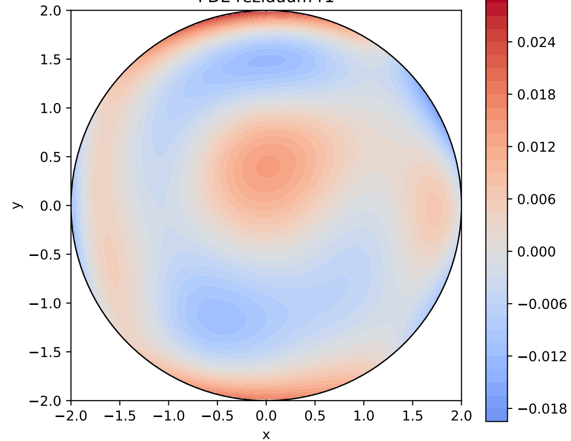
PDE reziduum r1
