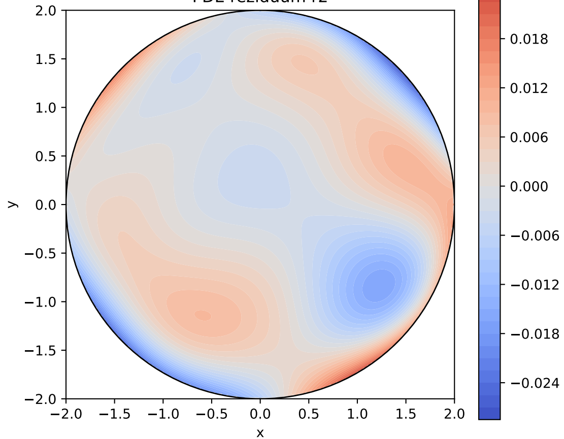
PDE reziduum r2
