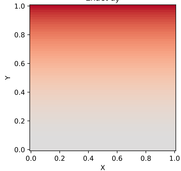
Exact u_y
