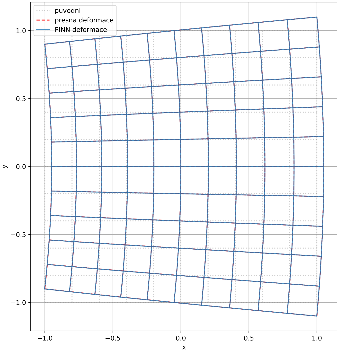
Deformovana oblast, meritko posunuti = 1.0
