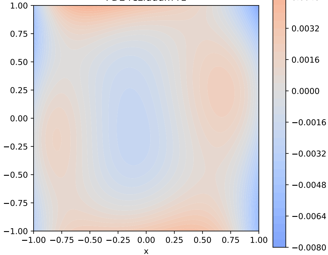
PDE reziduum r1
