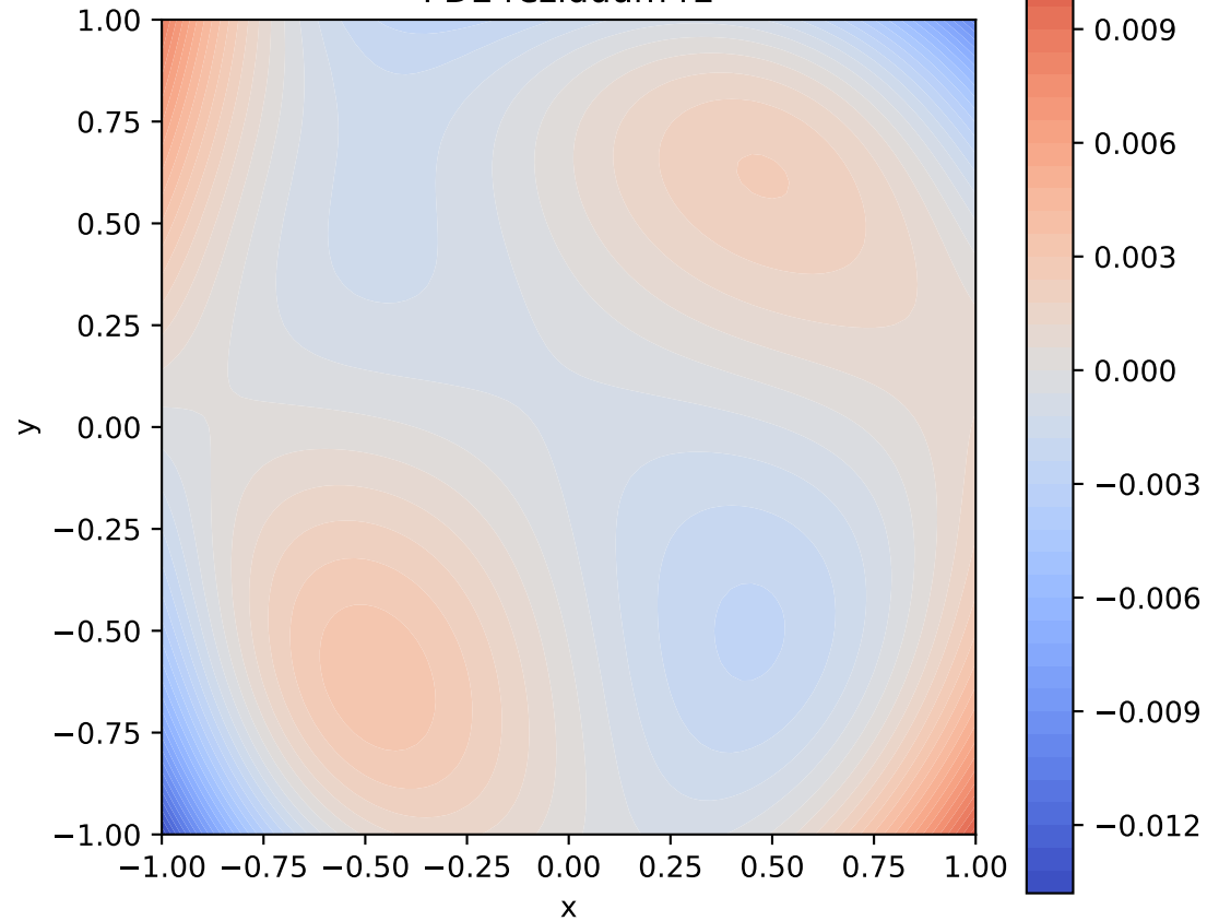
PDE reziduum r2
