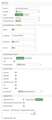
Fig. 6. Política de firewall "vpn_VPN_Lab_remote" (ravpn → port2).
