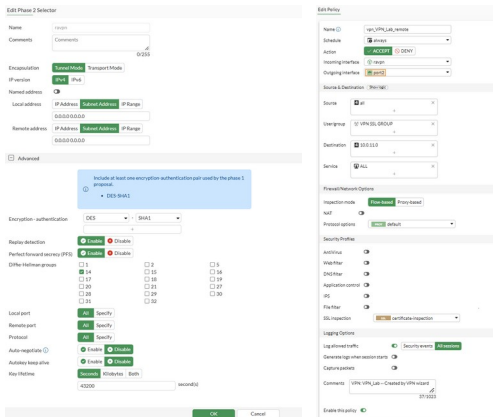
Fig. 4. Configuración del selector de Fase 2 del túnel "ravpn".
