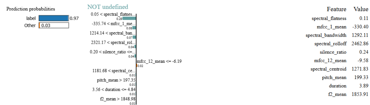
Figura 28: Explicación local de Random Forest con LIME
