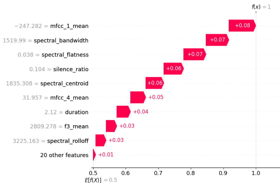
Figura 60: Explicación local de SVM con SHAP para audios nuevos en inglés
