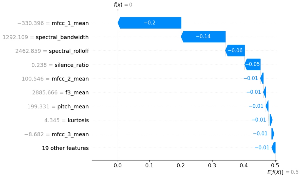
Figura 22: Explicación local de Random Forest con SHAP tras quitar spectral flatness
