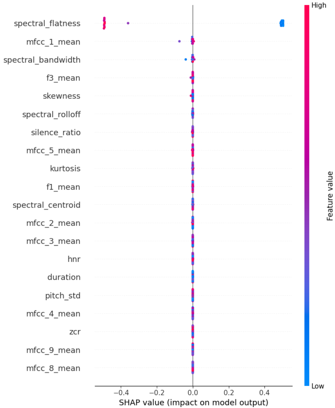
Figura 29: Explicación global de LightGBM con SHAP
