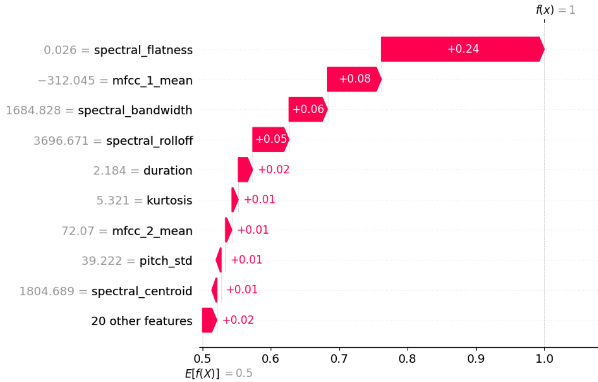
Figura 20: Explicación local de Random Forest con SHAP
