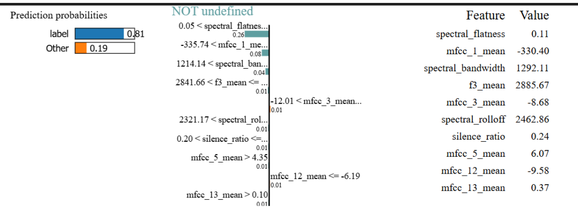
Figura 34: Explicación local de LightGBM con LIME
