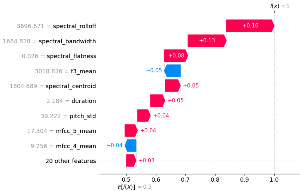
Figura 36: Explicación local de SVM con SHAP
