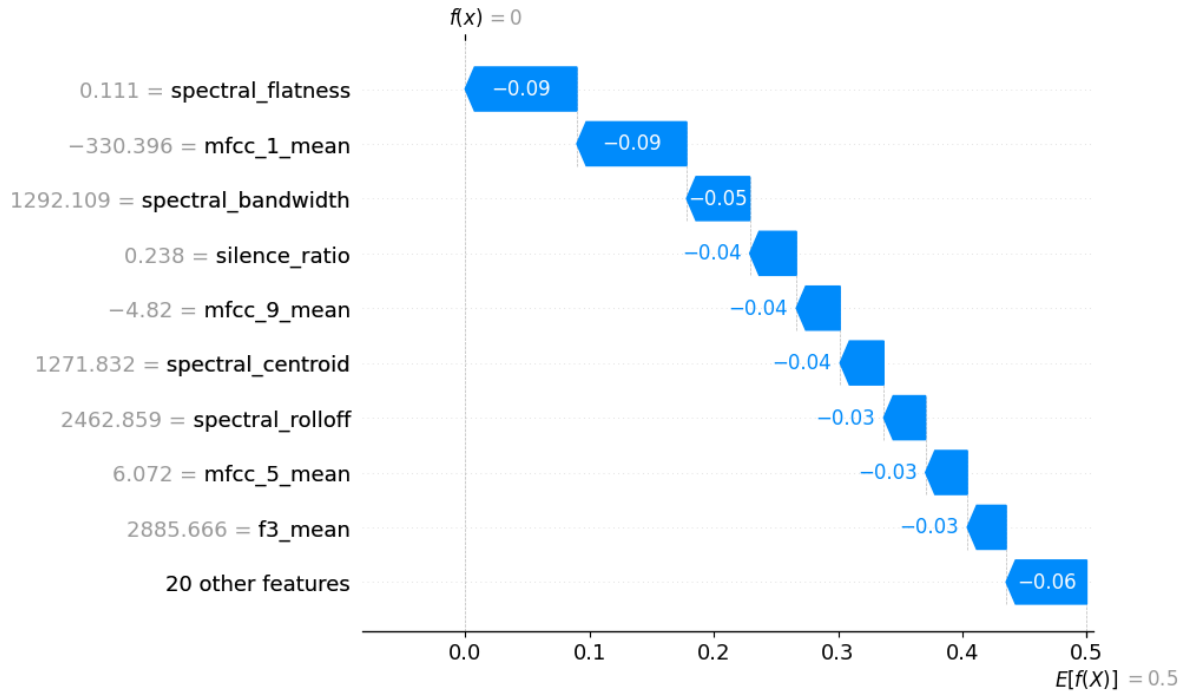
Figura 35: Explicación local de SVM con SHAP
