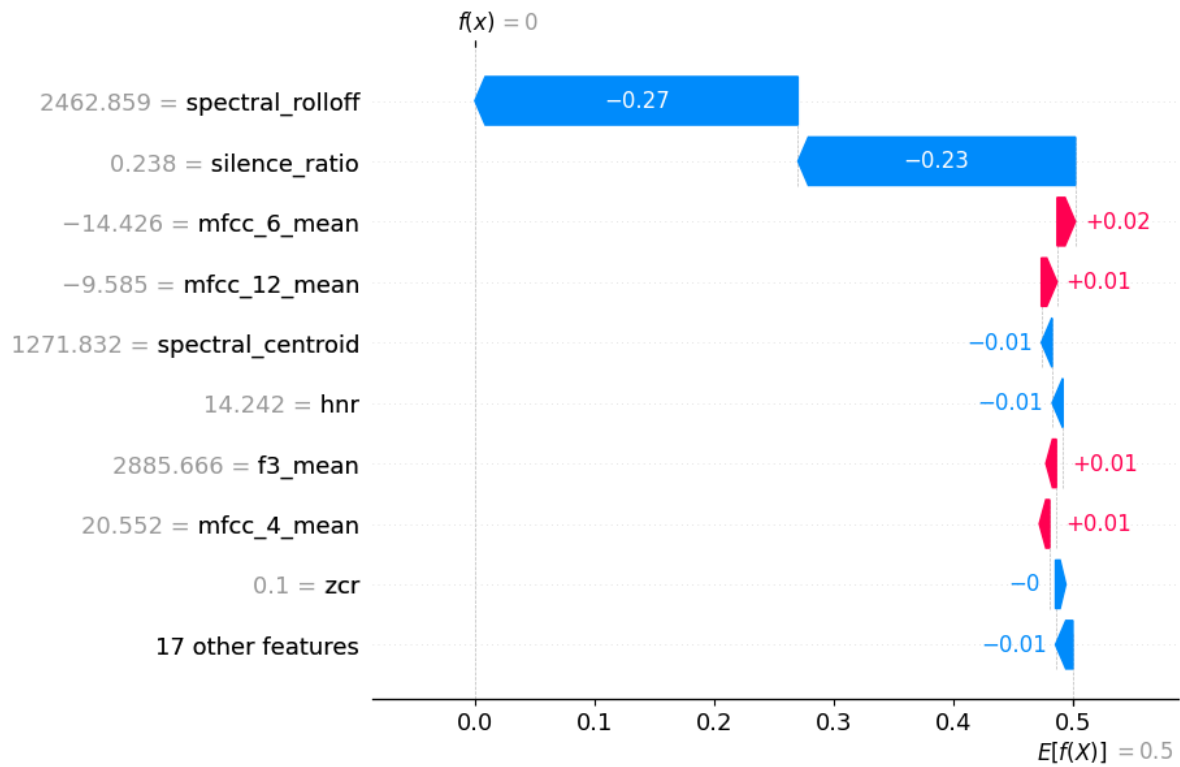
Figura 24: Explicación local de Random Forest con SHAP tras quitar spectral flatness, mfcc 1 y spectral bandwidth
