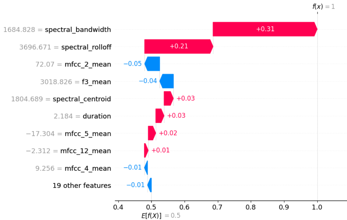
Figura 23: Explicación local de Random Forest con SHAP tras quitar spectral flatness
