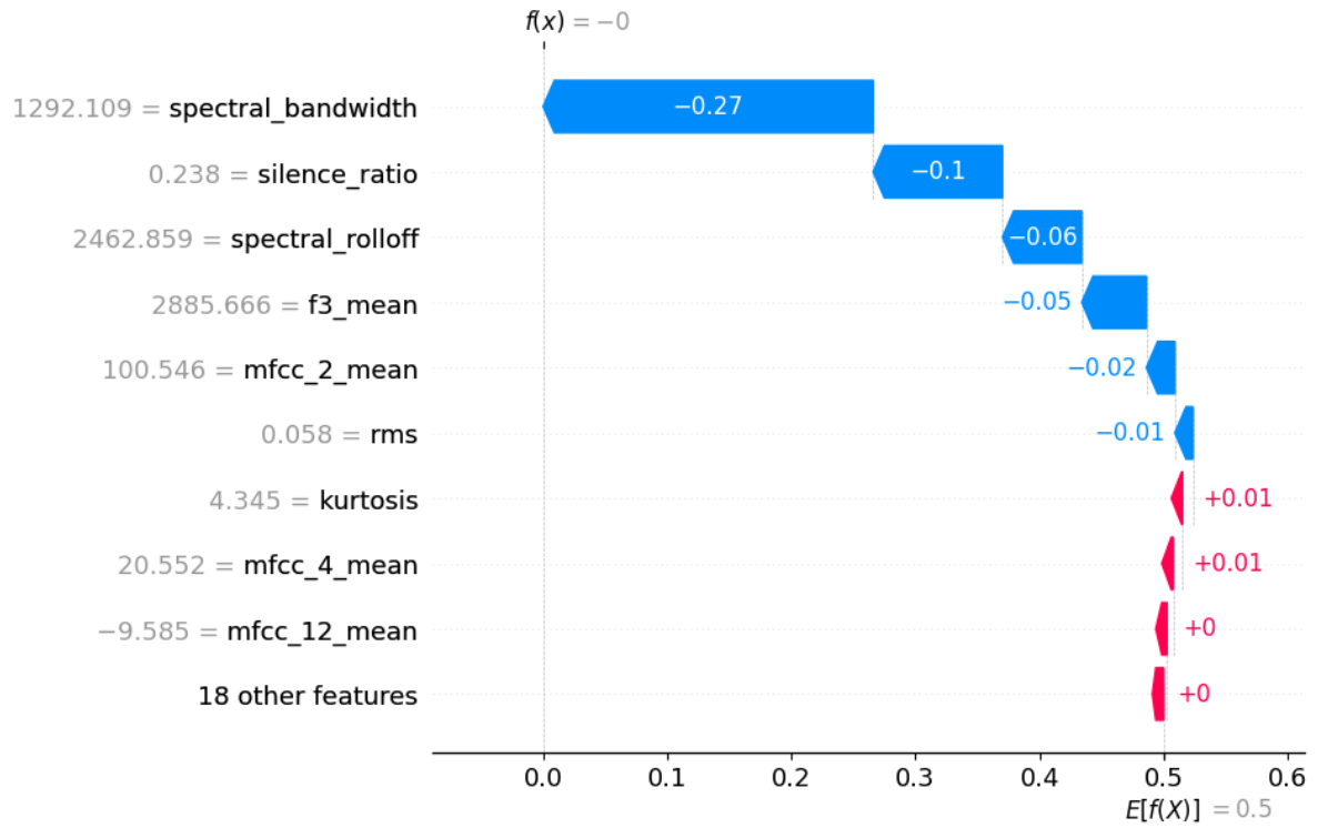
Figura 32: Explicación local de LightGBM con SHAP tras quitar spectral flatness y mfcc 1
