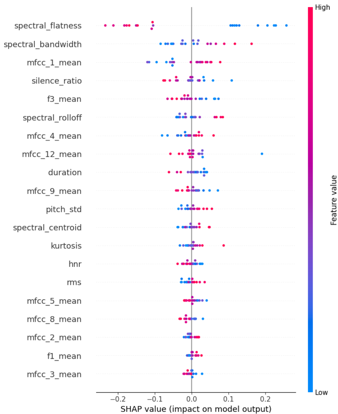
Figura 37: Explicación global de SVM con SHAP
