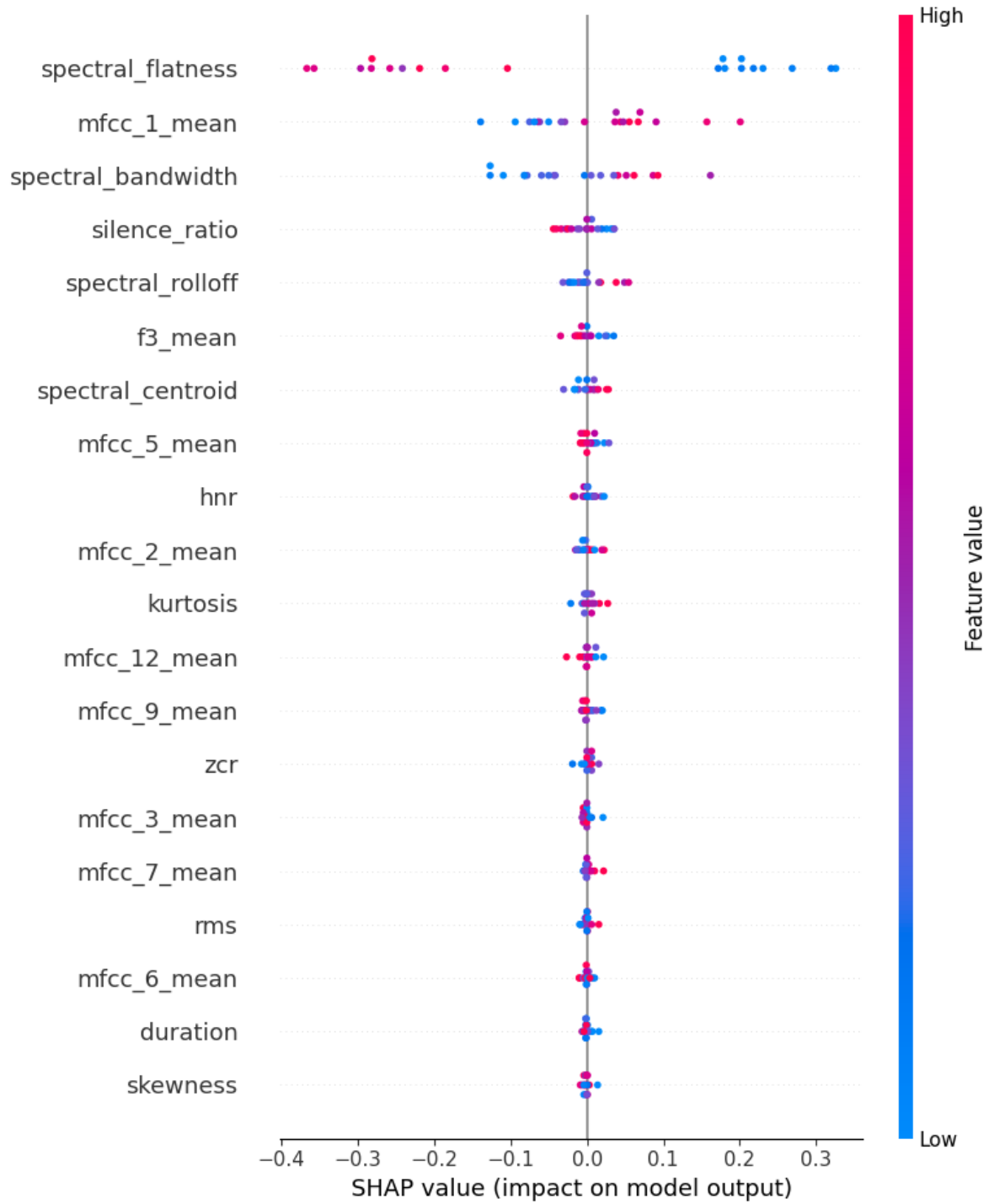
Figura 21: Explicación global de Random Forest con SHAP
