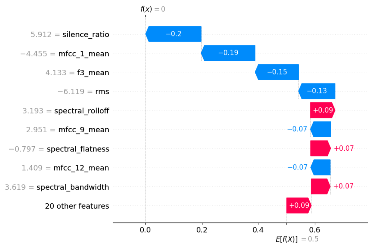
Figura 4.4: Explicación local de SHAP (Instancia 2) para el pipeline con KNN.
