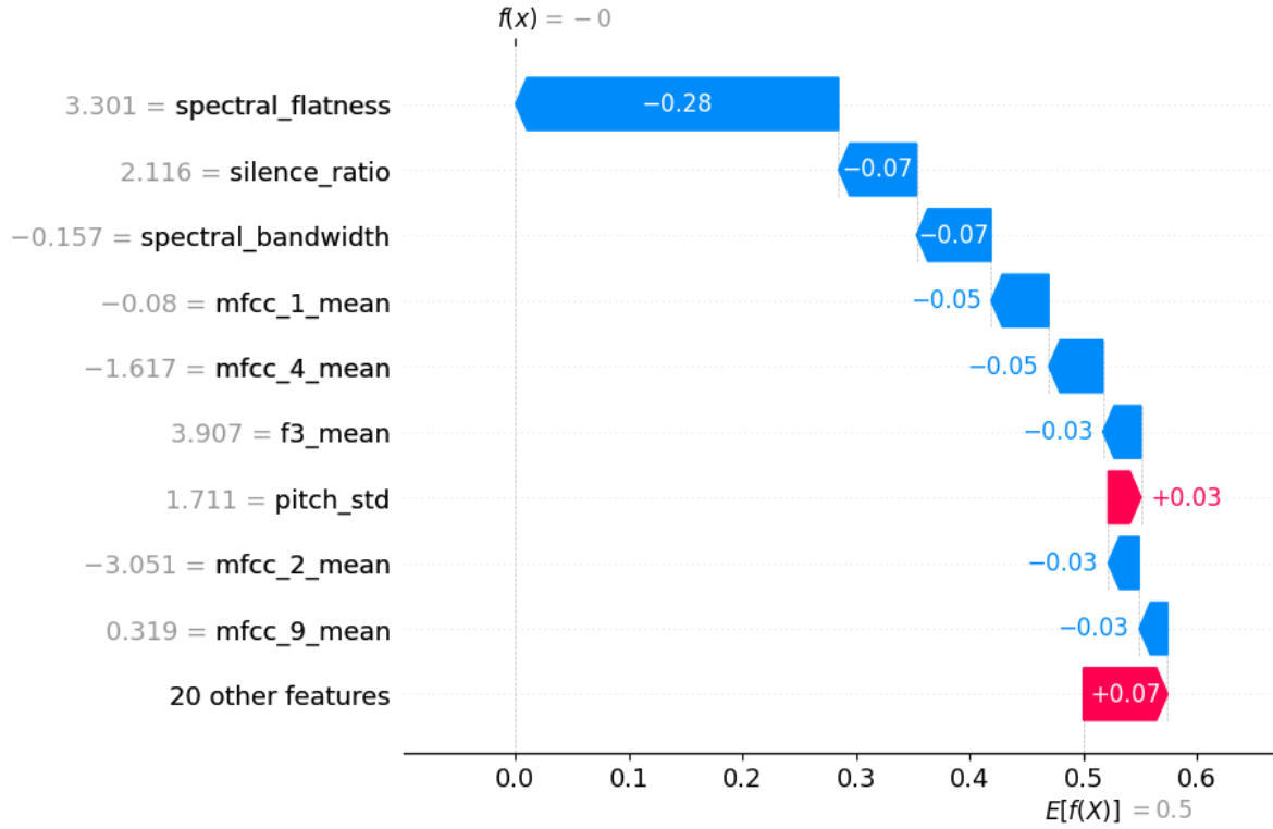
Figura 4.3: Explicación local de SHAP (Instancia 1) para el pipeline con KNN.
