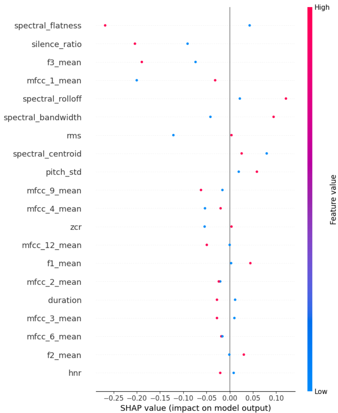
Figura 4.2: Importancia global de las características mediante SHAP para el pipeline con KNN.
