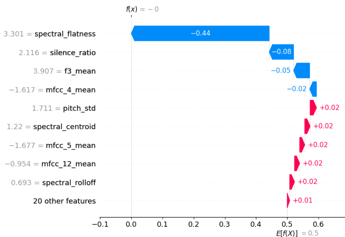
Figura 4.8: Explicación local de SHAP (Instancia 1) para el pipeline con Regresión Logística.
