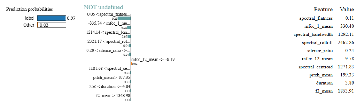
Figura 20: Explicación local de Random Forest con LIME
