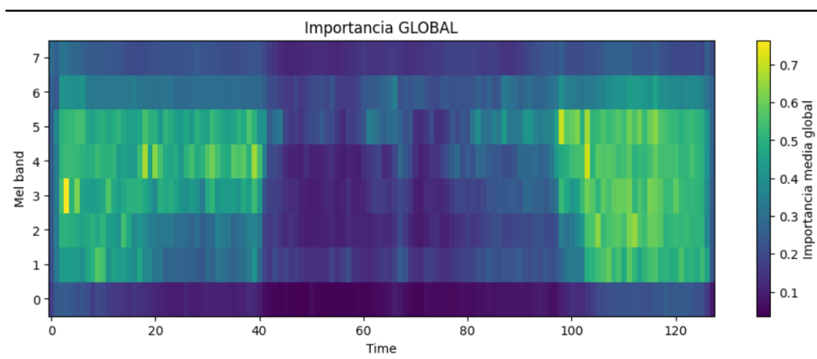
Figura 3.26: Influencia general de los espectrogramas
