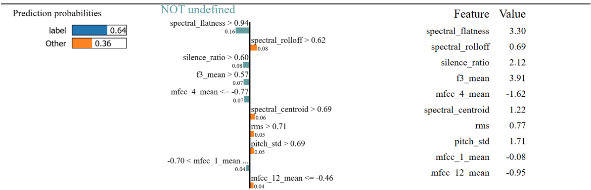
Figura 4.5: Explicación local de LIME (Instancia 1) para el pipeline con KNN.
