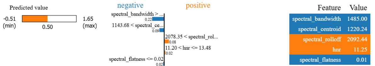
Figura 9: Explicación local espectrales Lime.
