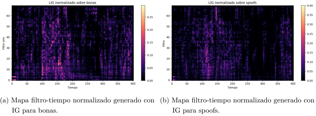
Figura 3.7: Mapas filtro-tiempo de la capa sinc-convolution generados con IG normalizados.
