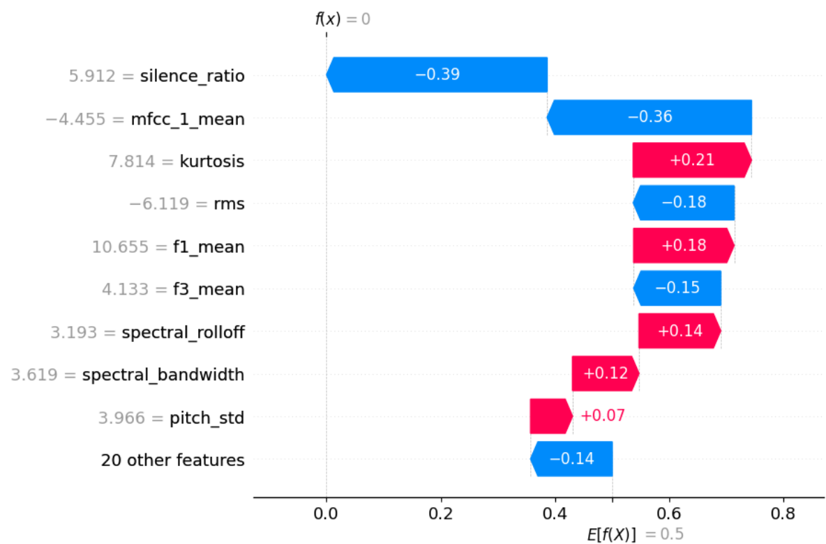
Figura 4.9: Explicación local de SHAP (Instancia 2) para el pipeline con Regresión Logística.
