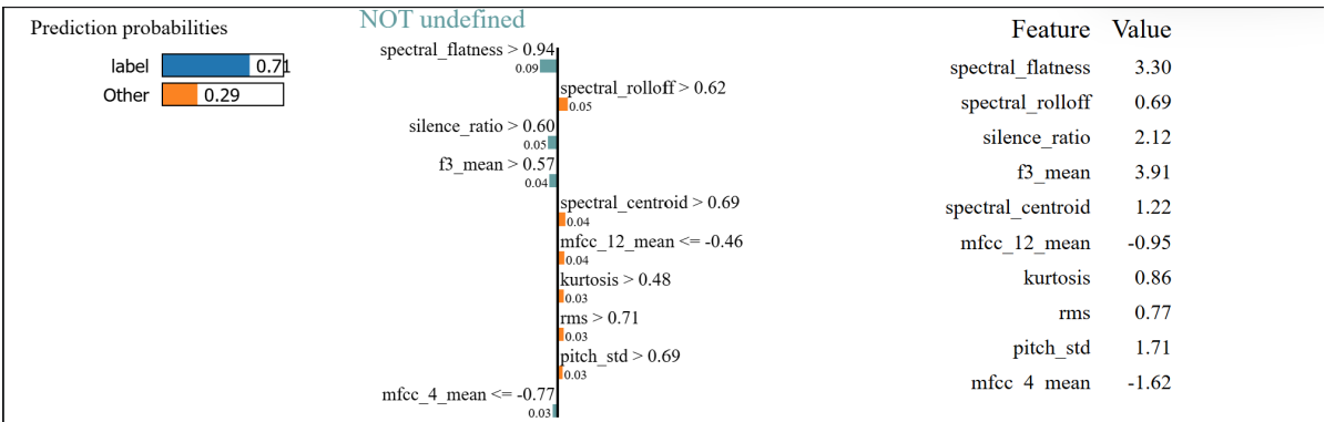
Figura 4.10: Explicación local de LIME (Instancia 1) para el pipeline con Regresión Logística.
