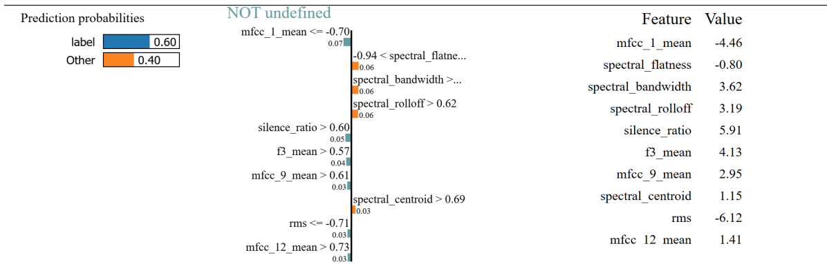
Figura 4.11: Explicación local de LIME (Instancia 2) para el pipeline con Regresión Logística.
