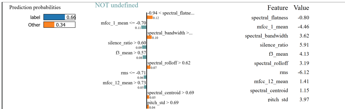
Figura 4.6: Explicación local de LIME (Instancia 2) para el pipeline con KNN.
