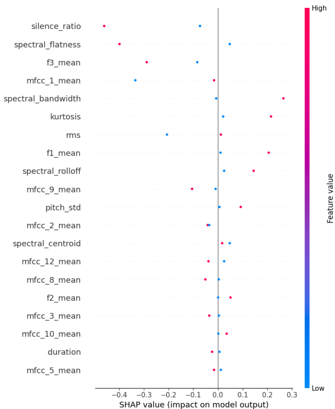
Figura 4.7: Importancia global de las características mediante SHAP para el pipeline con Regresión Logística.
