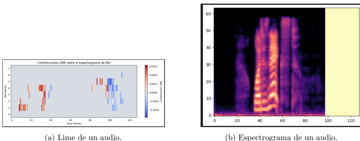
Figura 3.20: Lime local sobre los espectrogramas con Wav2Vec2
