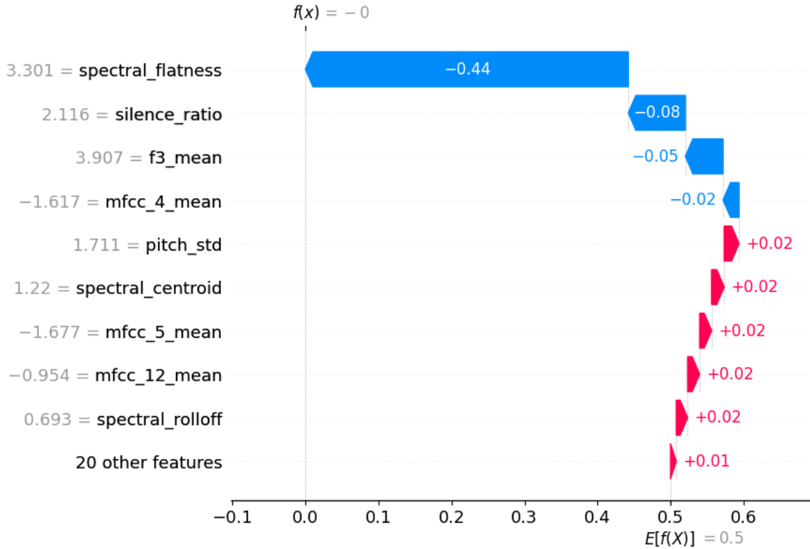
Figura 4.8: Explicación local de SHAP (Instancia 1) para el pipeline con Regresión Logística.
