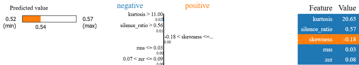
Figura 3.20: Explicación local energía Lime.
