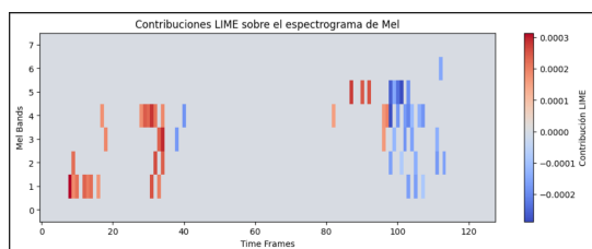
(a) Lime de un audio.
