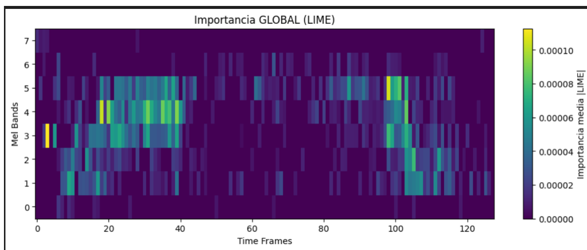
Figura 3.36: Lime general de los espectrogramas
