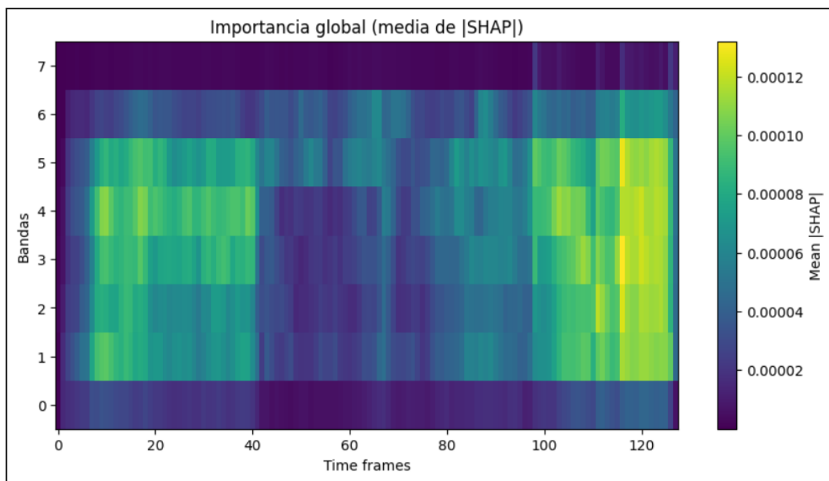
Figura 3.34: Shap general de los espectrogramas
