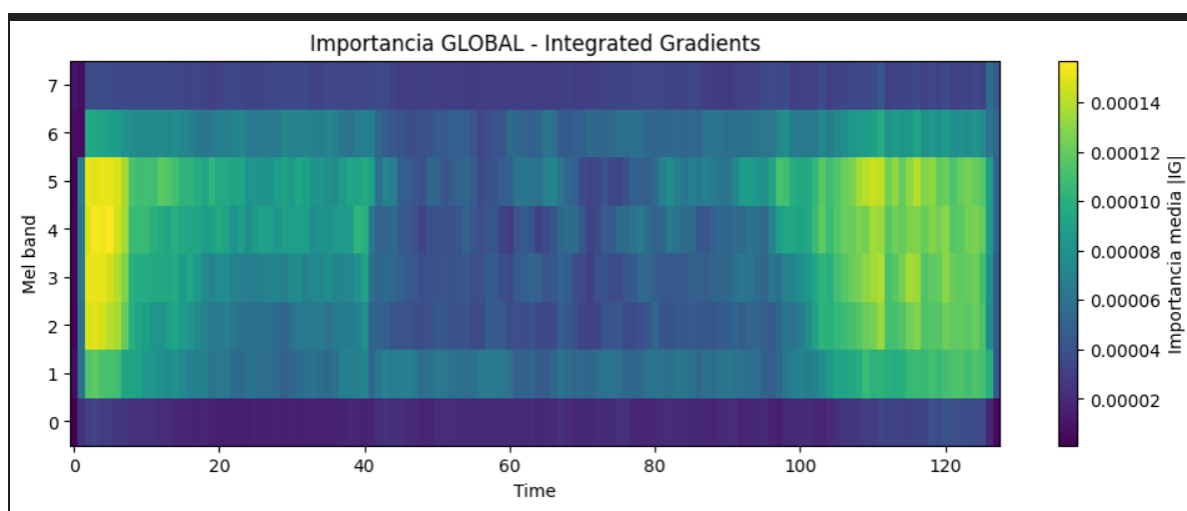
Figura 3.13: Integrated gradients general de los espectrogramas
