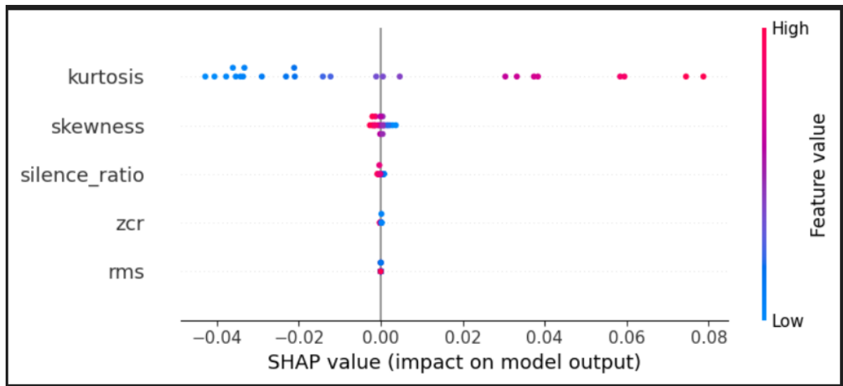
Figura 3.12: Shap global energía.
