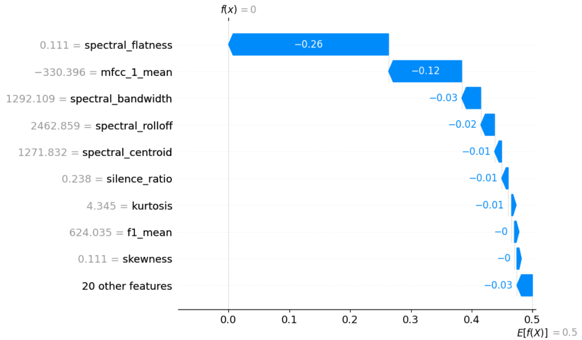
Figura 13: Explicación local de Random Forest con SHAP
