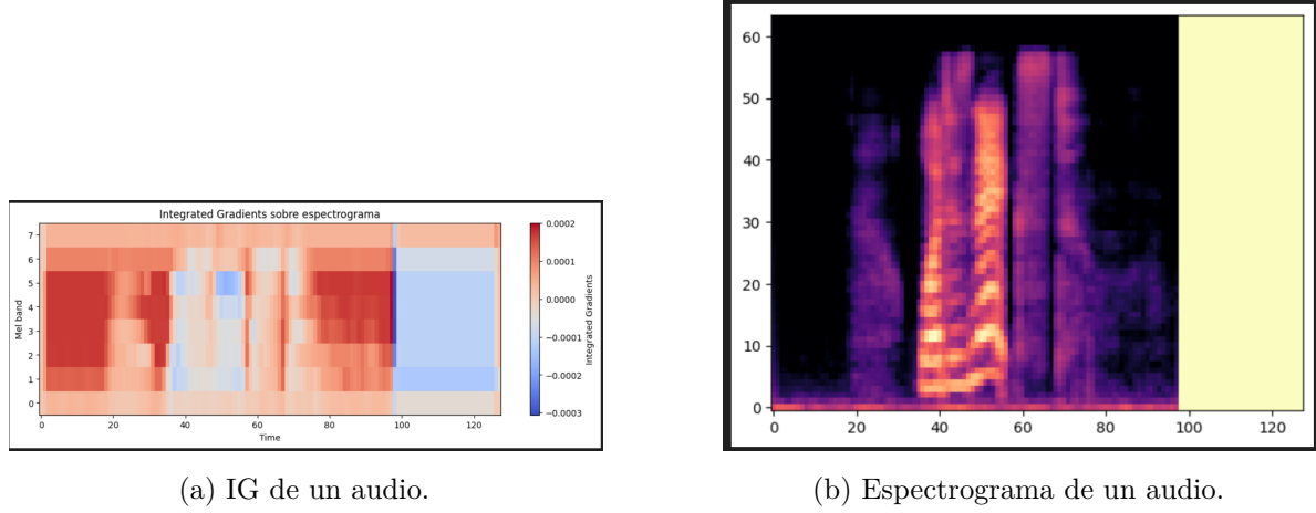
Figura 3.37: IG local espectrogramas Wav2Vec2
