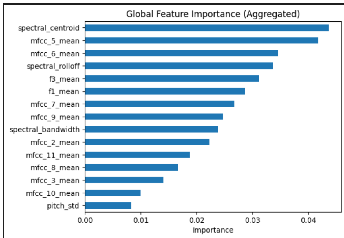
Figura 3.30: Ranking características Shap.
