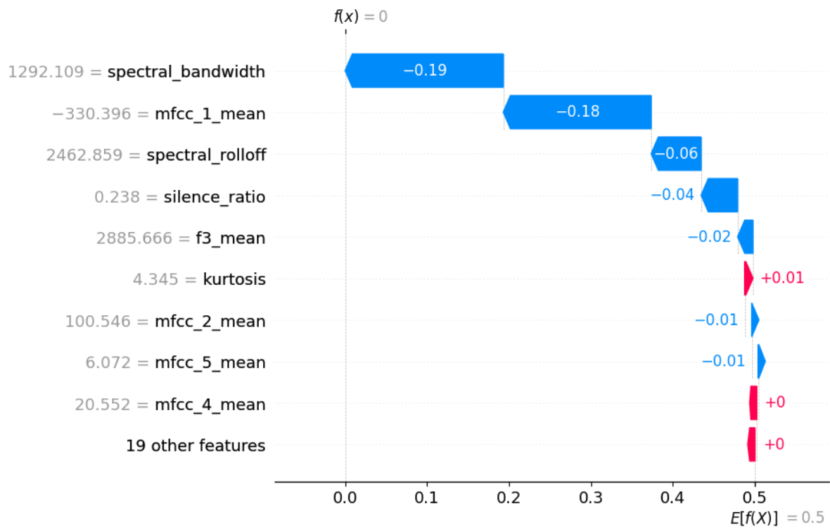
Figura 31: Explicación local de LightGBM con SHAP tras quitar spectral flatness
