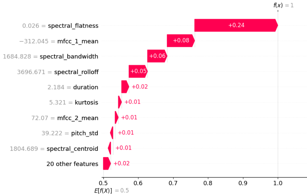
Figura 21: Explicación local de Random Forest con SHAP
