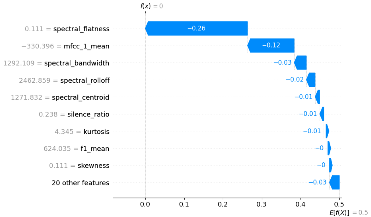
Figura 20: Explicación local de Random Forest con SHAP
