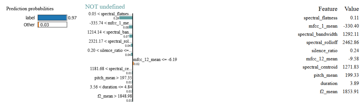
Figura 27: Explicación local de Random Forest con LIME
