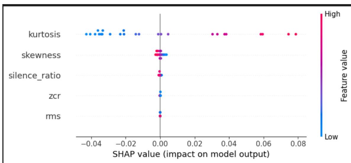
Figura 3.3: Shap global energía.
