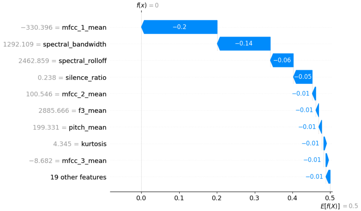
Figura 23: Explicación local de Random Forest con SHAP tras quitar spectral flatness
