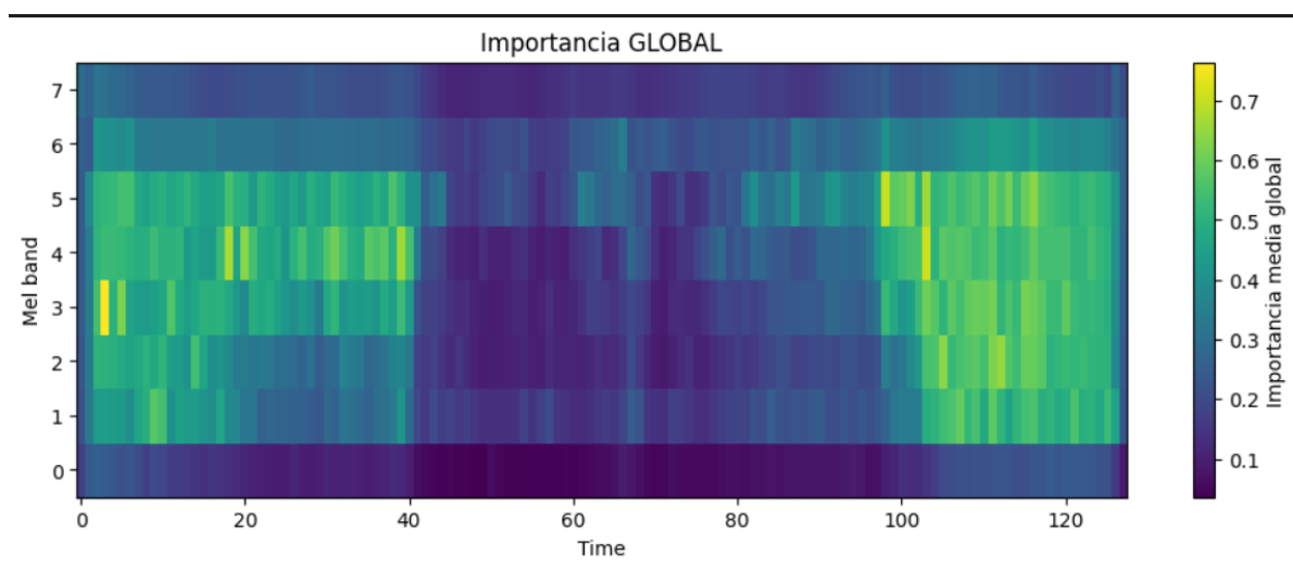
Figura 3.17: Influencia general de los espectrogramas
