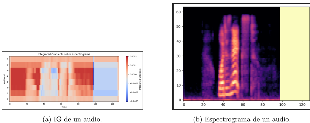
Figura 3.13: IG local espectrogramas Wav2Vec2
