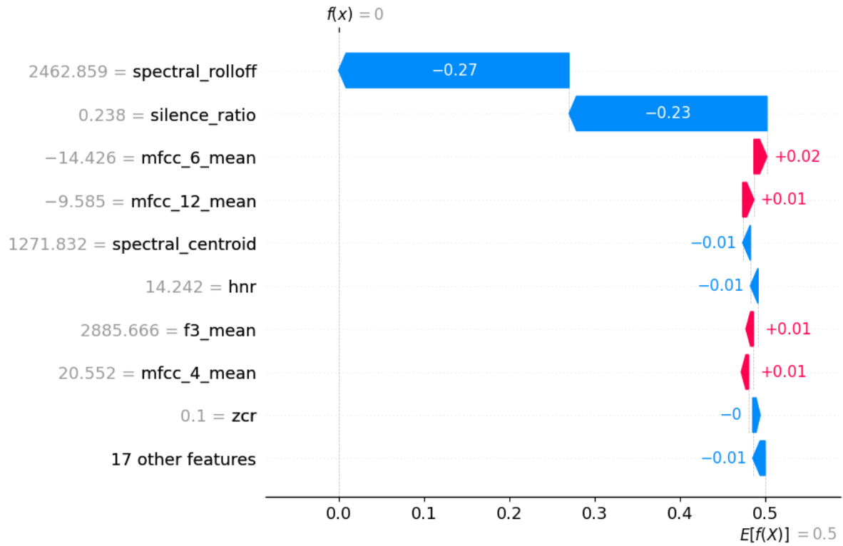
Figura 25: Explicación local de Random Forest con SHAP tras quitar spectral flatness, mfcc 1 y spectral bandwidth
