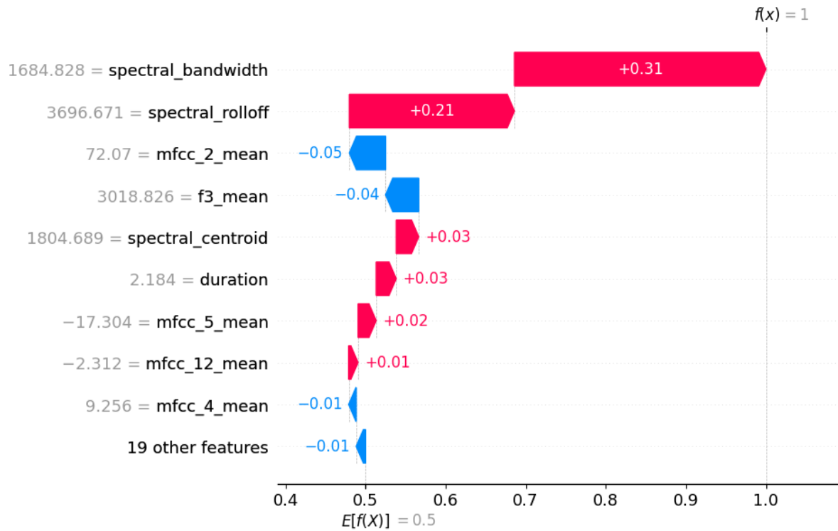
Figura 24: Explicación local de Random Forest con SHAP tras quitar spectral flatness
