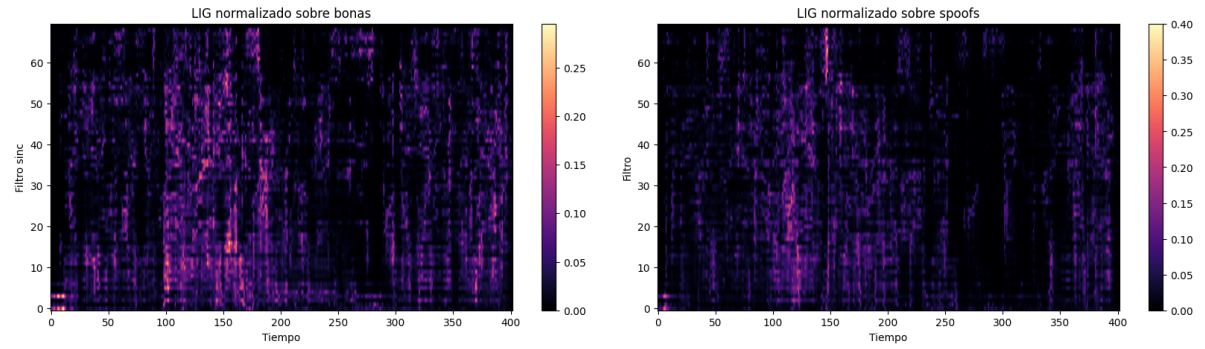
Figura 5: Mapas filtro-tiempo de la capa sinc-convolution generados con IG.
