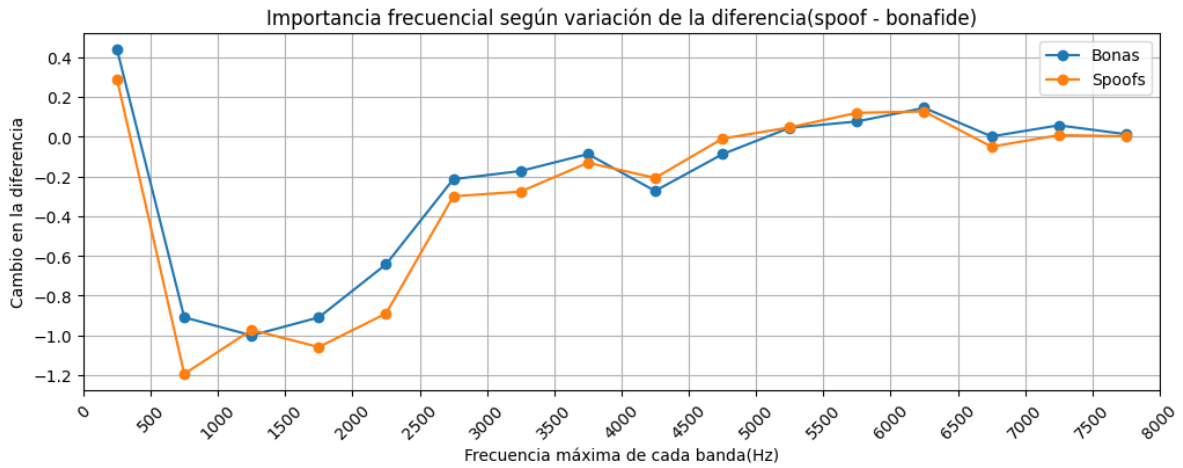
Figura 4: Resultados de margen de la ocultación frecuencial en AASIST.
