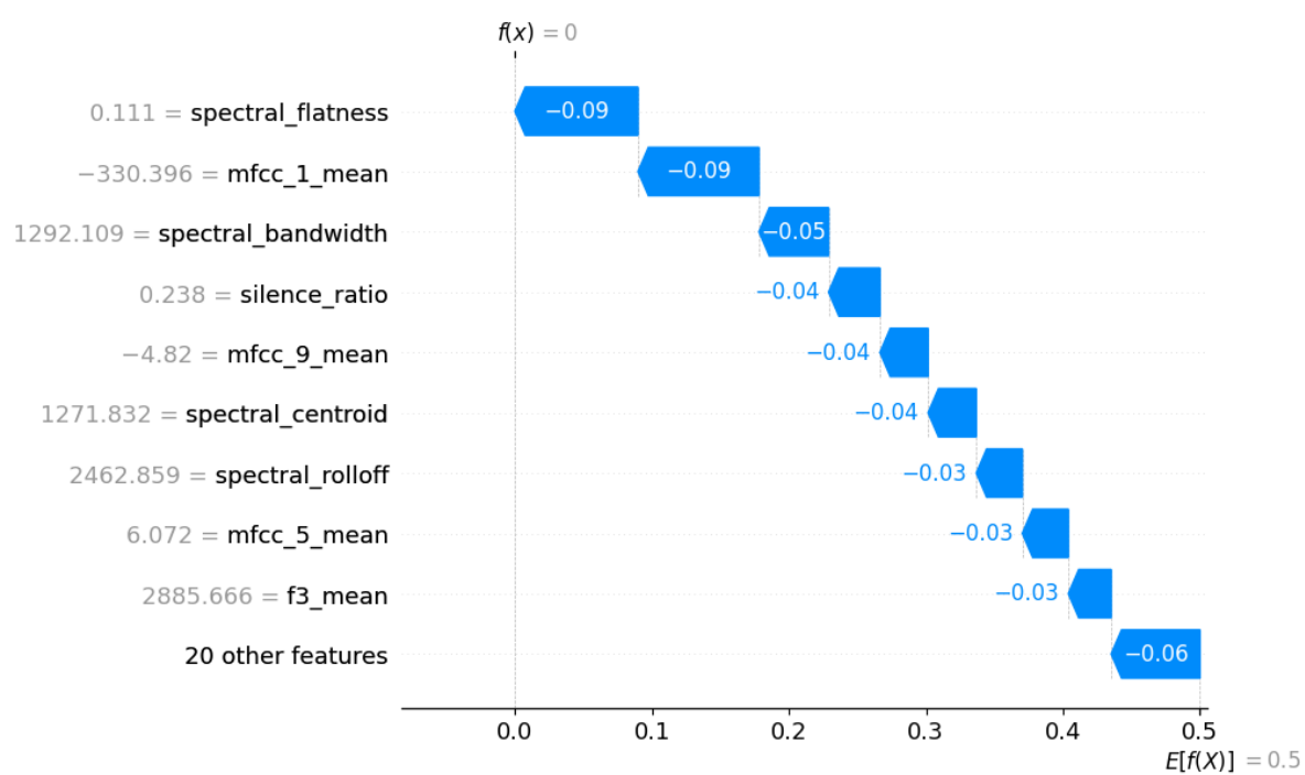
Figura 36: Explicación local de SVM con SHAP
