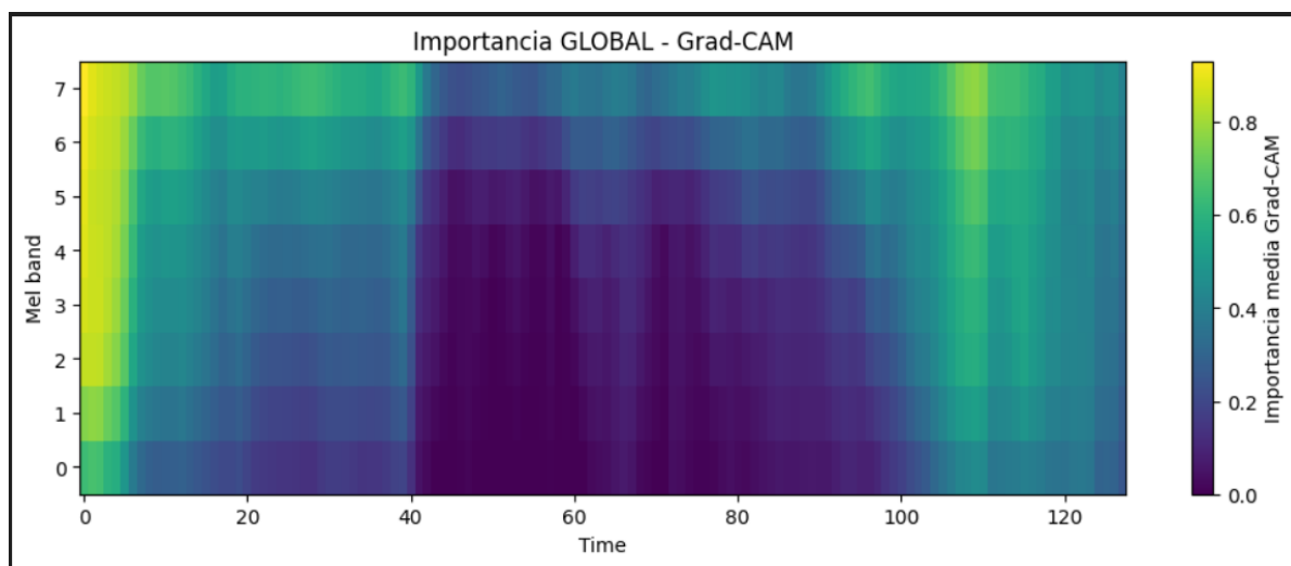
Figura 3.16: Grad cam general de los espectrogramas
