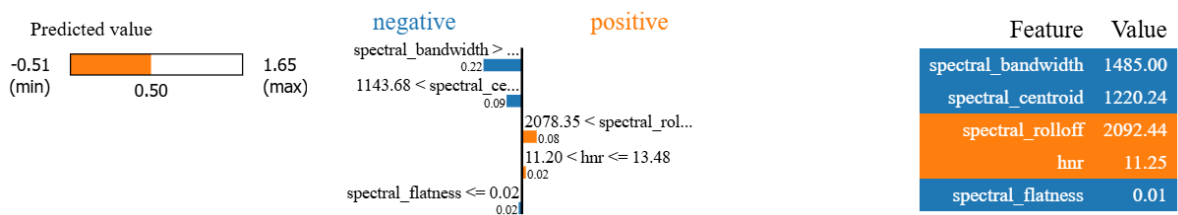
Figura 9: Explicación local espectrales Lime.
