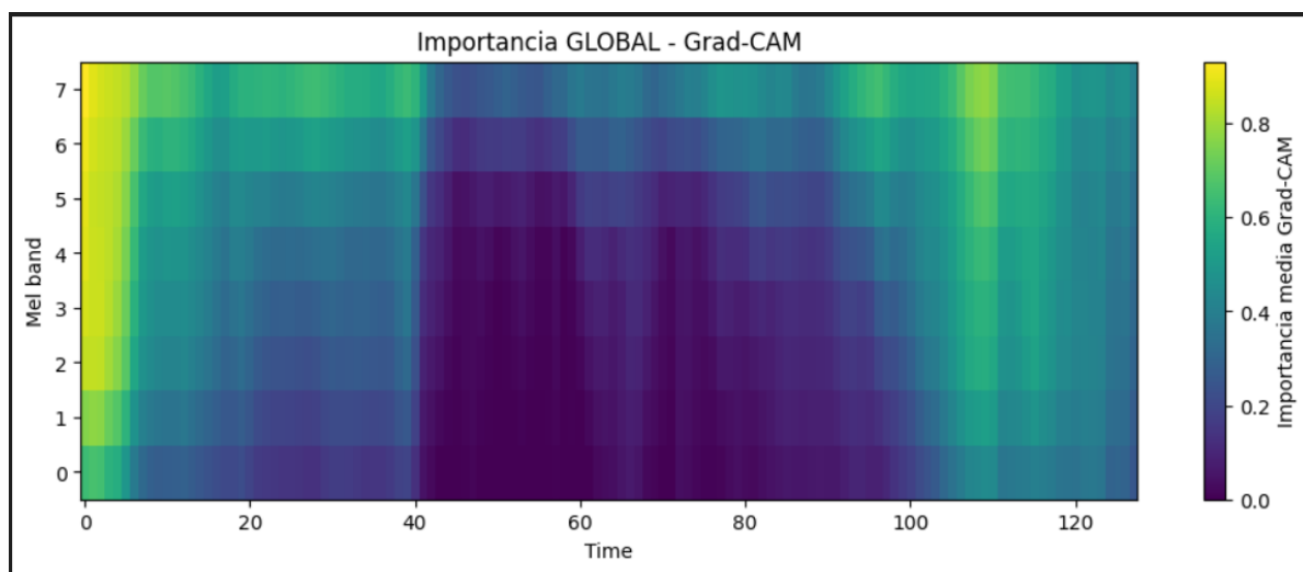
Figura 3.25: Grad Cam general de los espectrogramas
