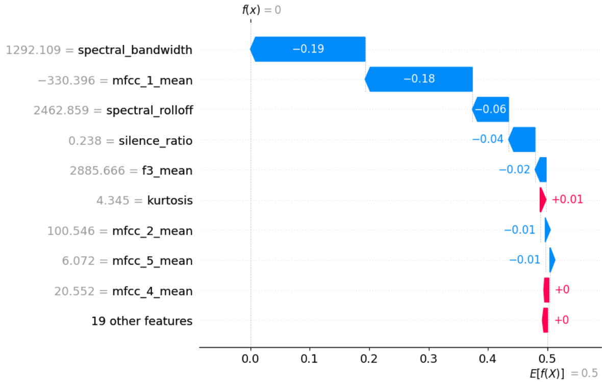
Figura 24: Explicación local de LightGBM con SHAP tras quitar spectral flatness
