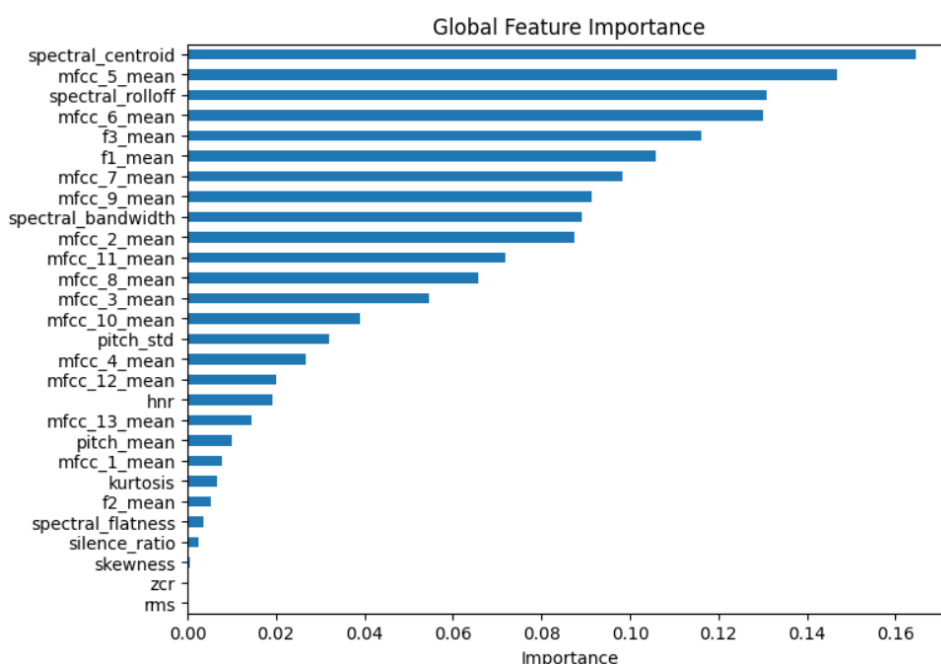
Figura 3.17: Ranking agregado de características.
