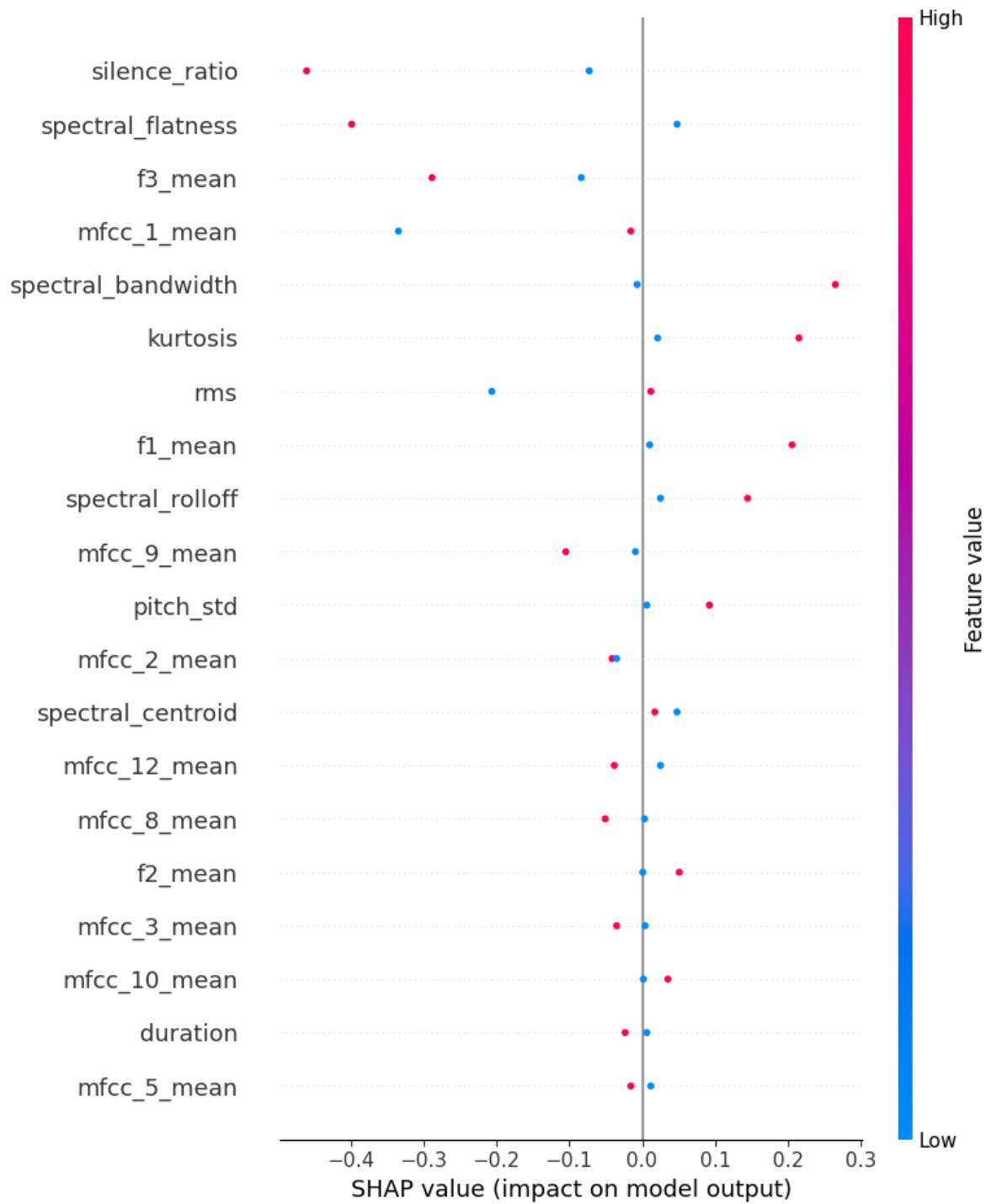
Figura 70: Importancia global de las características mediante SHAP para el pipeline con Regresión Logística.
