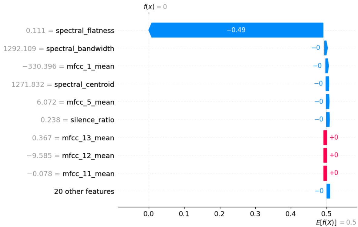
Figura 21: Explicación local de LightGBM con SHAP
