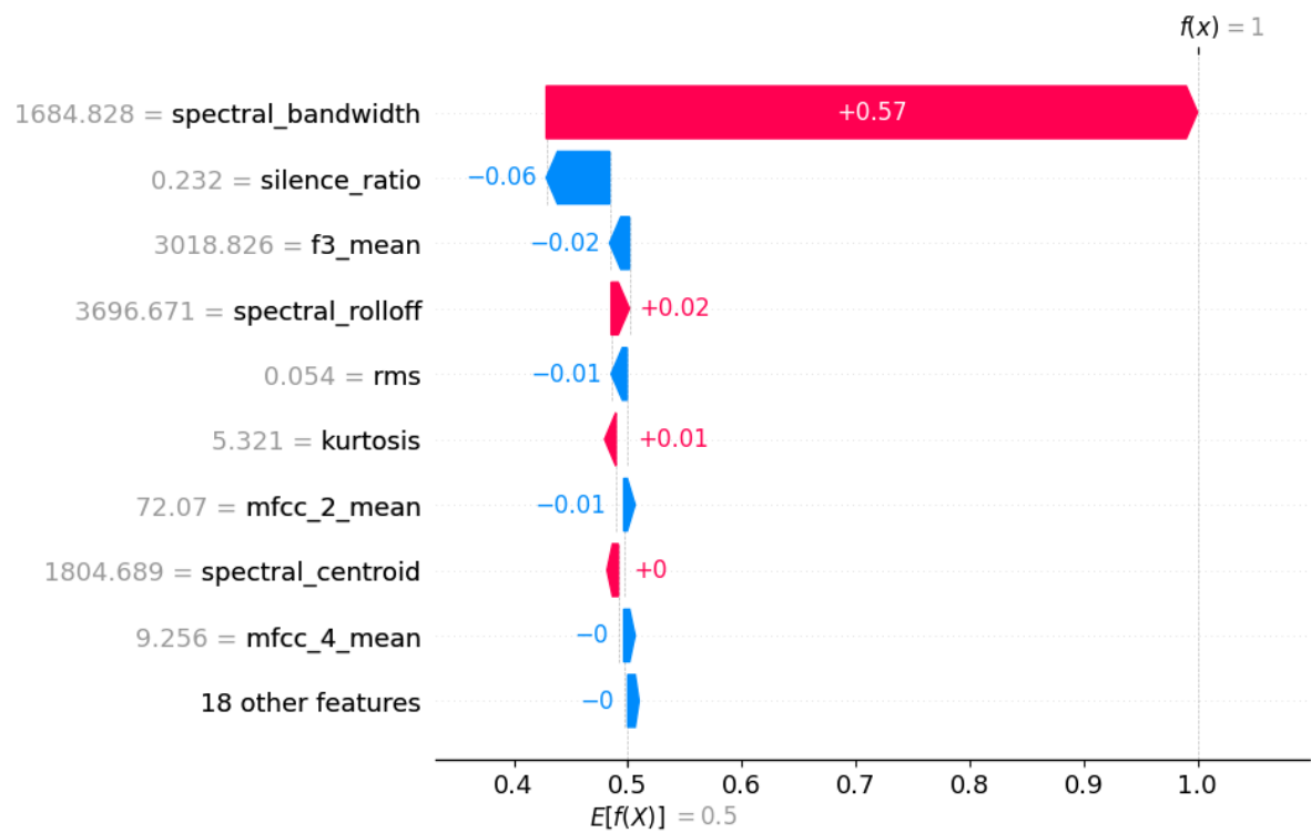
Figura 27: Explicación local de LightGBM con SHAP tras quitar spectral flatness y mfcc 1
