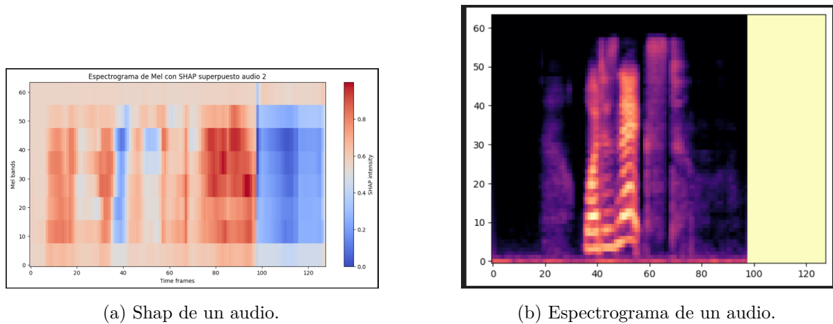
Figura 3.24: shap local espectrogramas Wav2Vec2
