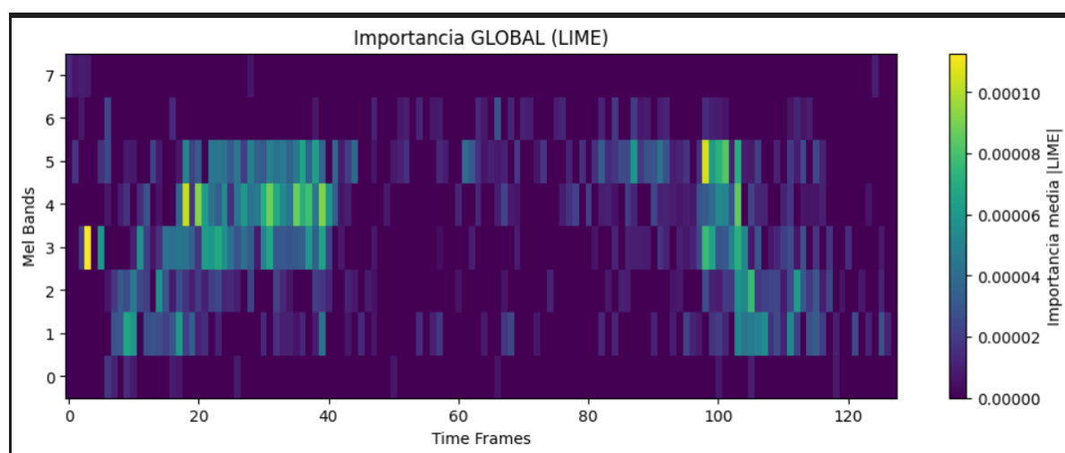
Figura 3.27: Lime general de los espectrogramas
