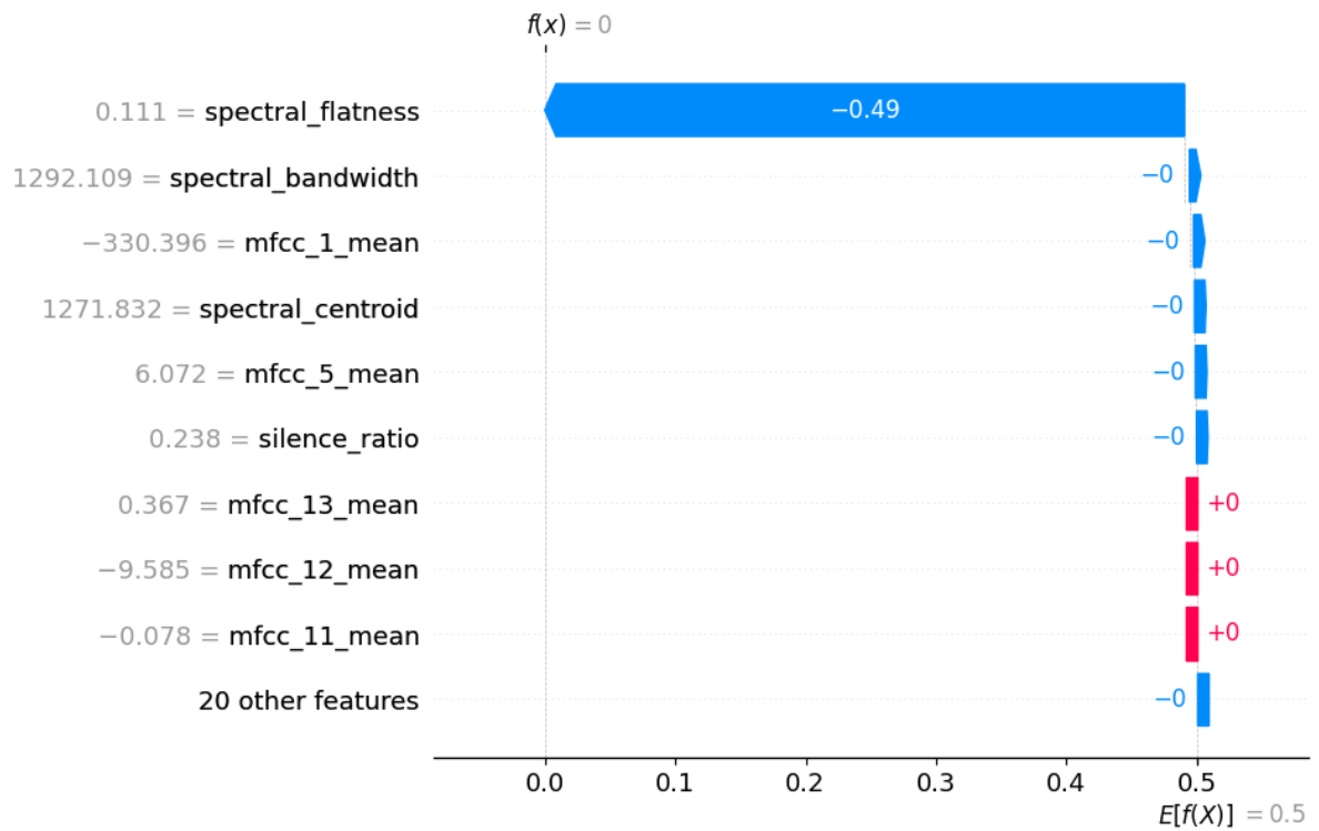
Figura 29: Explicación local de LightGBM con SHAP
