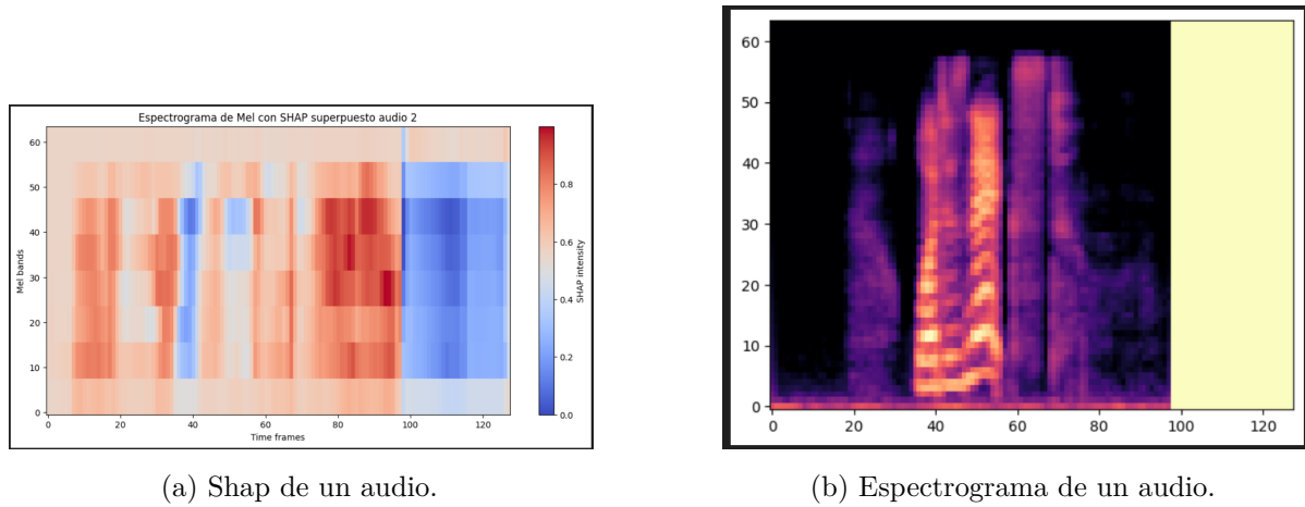
Figura 3.8: shap local espectrogramas Wav2Vec2
