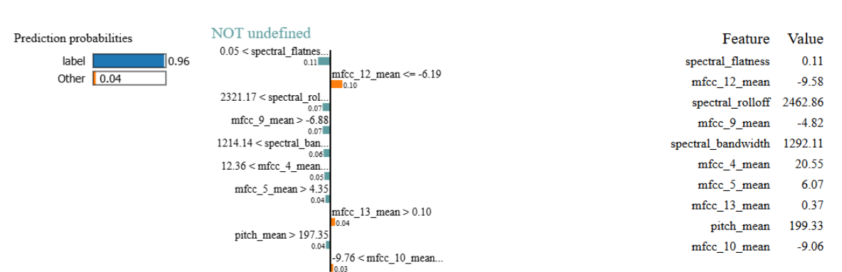
Figura 3.25: Explicación local con LIME
