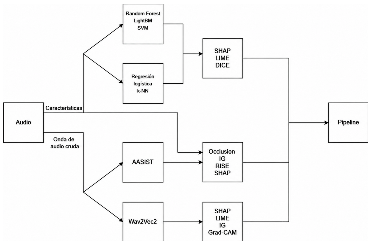
Figura 4.1: Arquitectura del pipeline.
