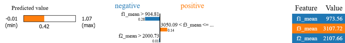
Figura 11: Explicación local formantes Lime.
