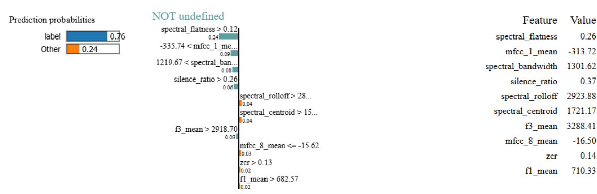
Figura 42: Explicación local de RF con LIME
