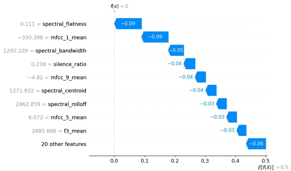
Figura 29: Explicación local de SVM con SHAP
