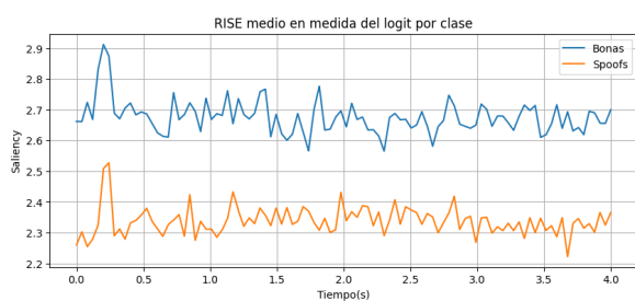
(a) Resultados de logit usando RISE.
