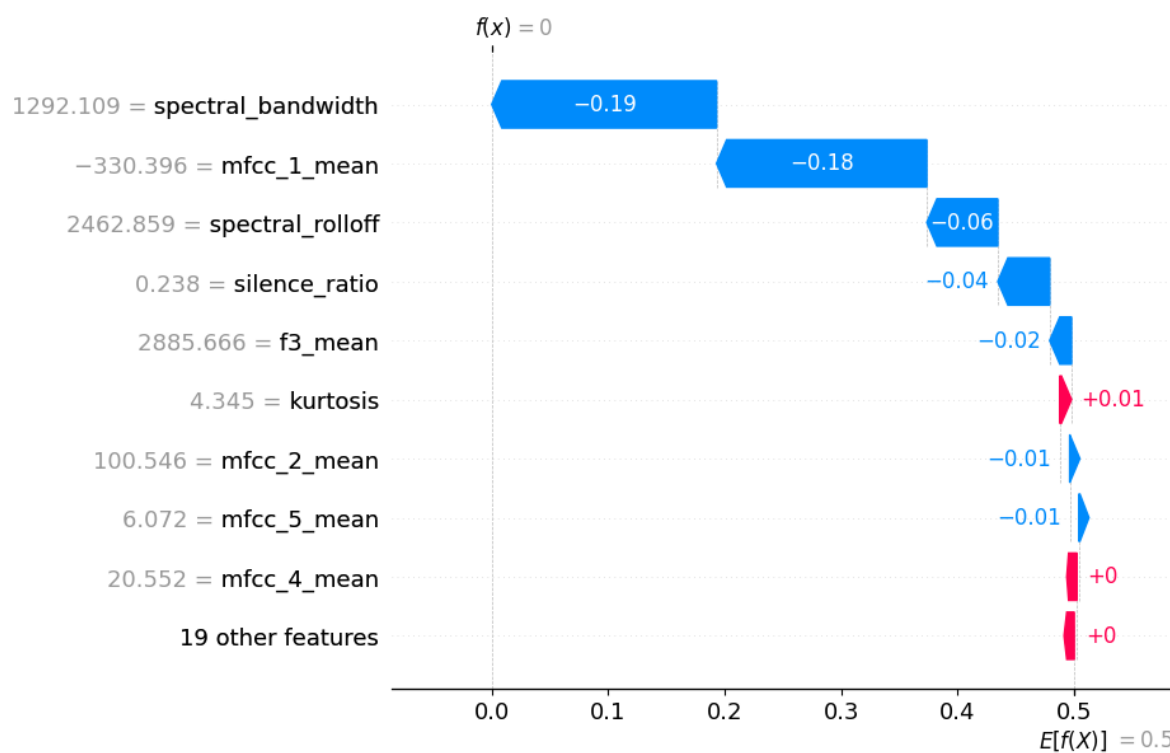
Figura 3.13: Explicación local con SHAP tras quitar spectral flatness
