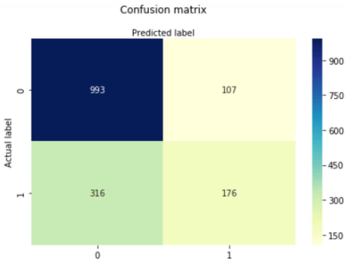
Figura 3.1: Ejemplo real de matriz de confusión.
