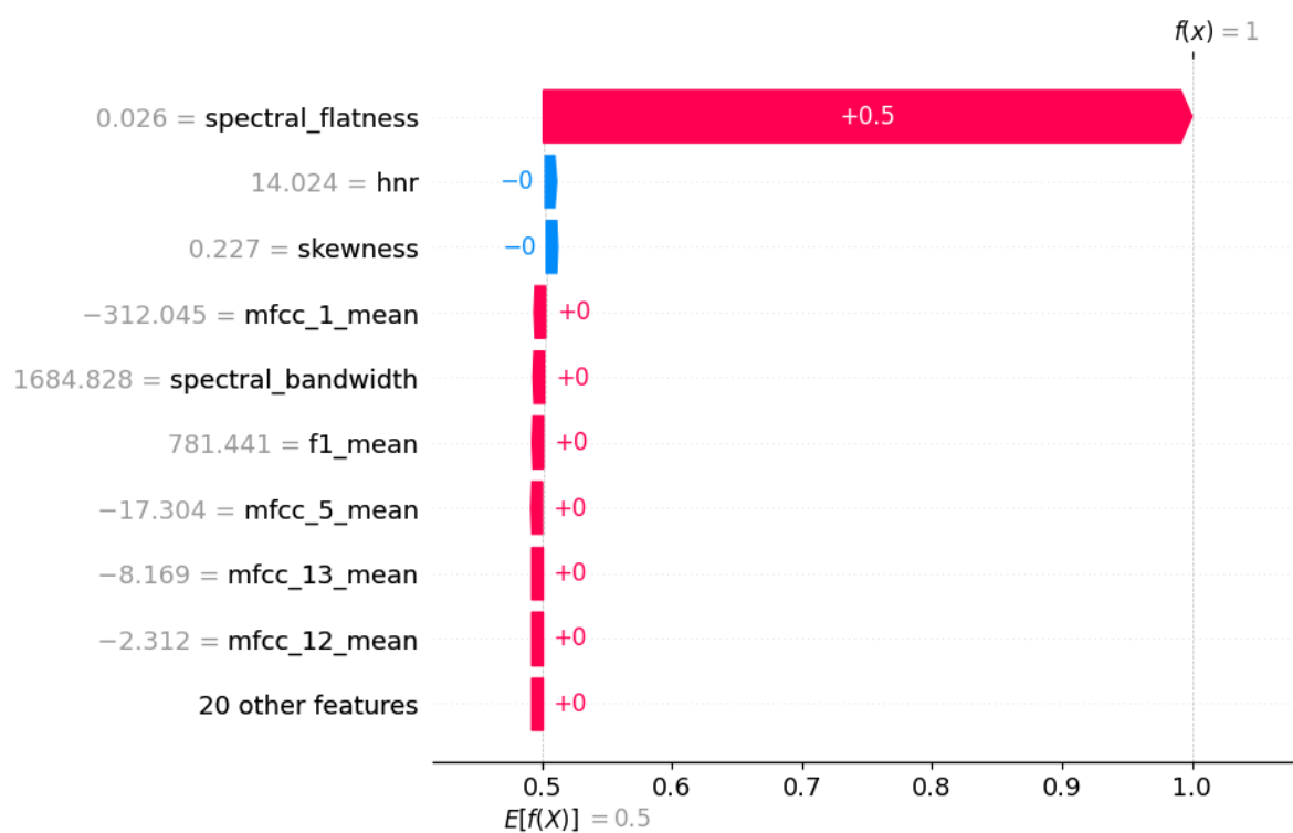
Figura 3.11: Explicación local con SHAP
