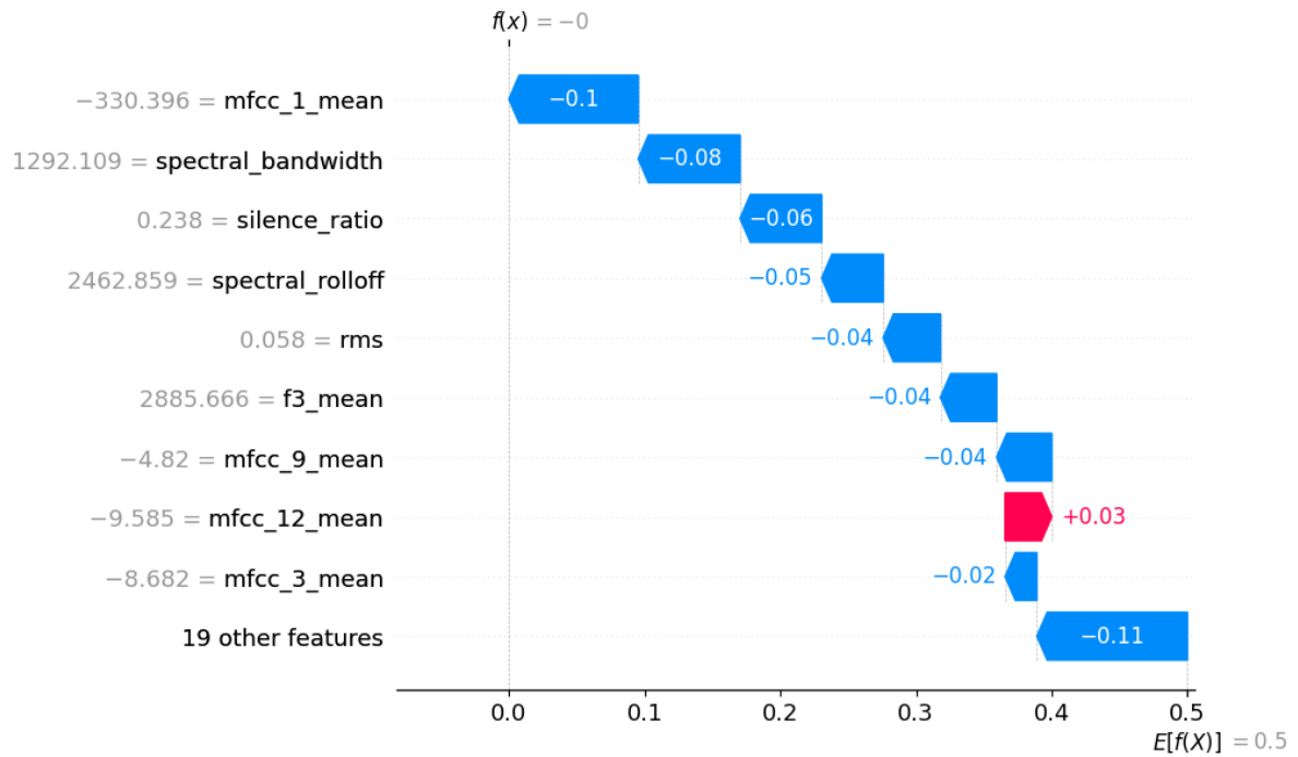
Figura 3.21: Explicación local con SHAP tras quitar spectral flatness
