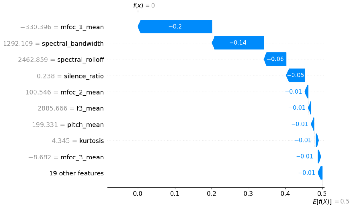
Figura 3.5: Explicación local con SHAP tras quitar spectral flatness
