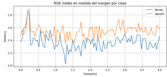
(b) Resultados de “margin” usando RISE.
