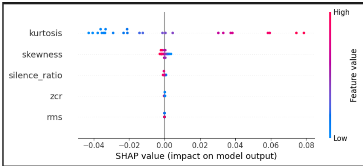
Figura 3.27: Shap global energía.
