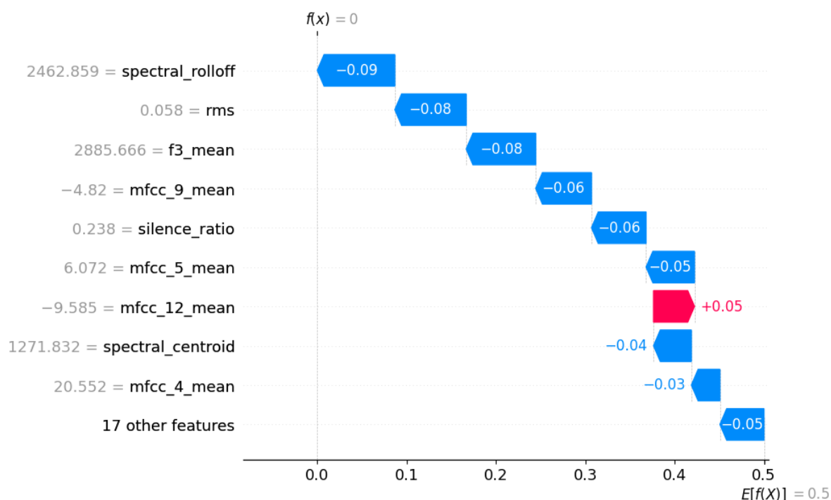
Figura 3.23: Explicación local con SHAP tras quitar spectral flatness, mfcc 1 y spectral bandwidth
