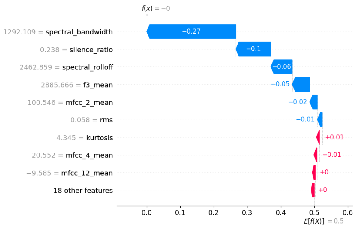
Figura 3.15: Explicación local con SHAP tras quitar spectral flatness y mfcc 1
