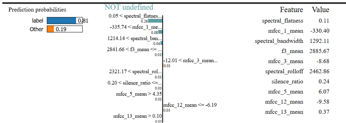
Figura 3.17: Explicación local con LIME
