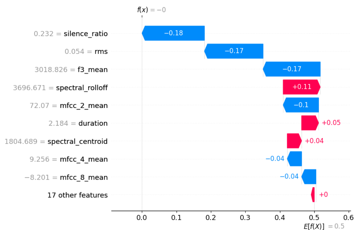
Figura 3.8: Explicación local con SHAP tras quitar spectral flatness, mfcc 1 y spectral bandwidth
