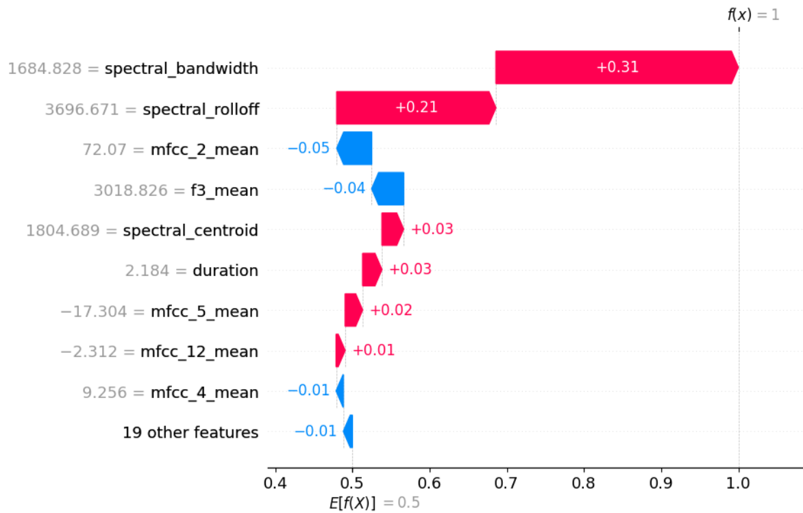
Figura 3.6: Explicación local con SHAP tras quitar spectral flatness
