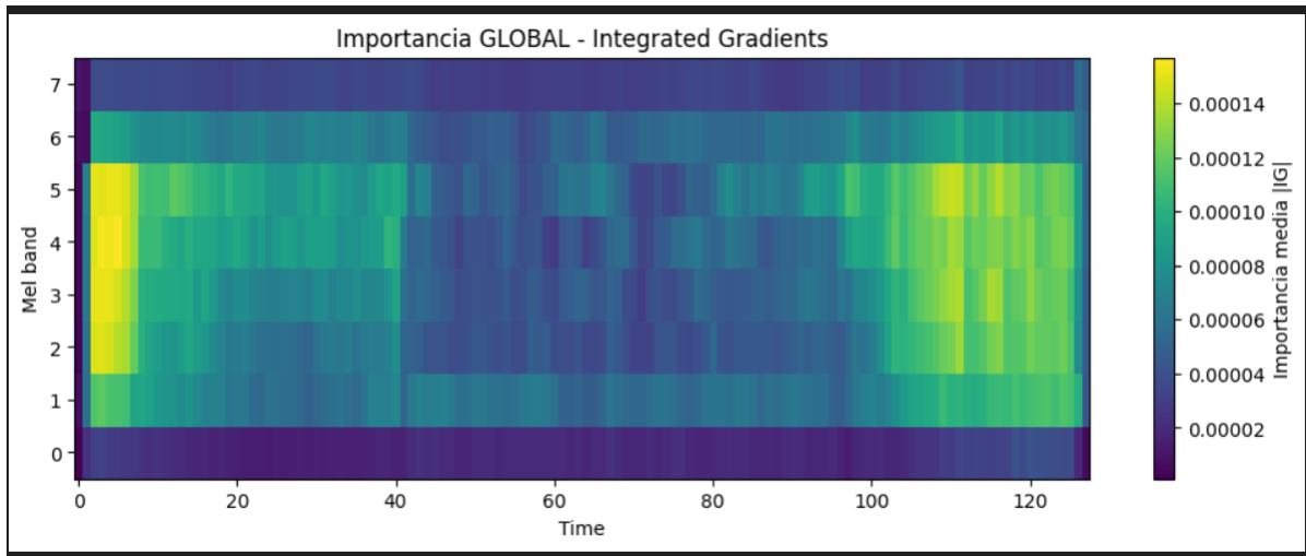
Figura 3.38: Integrated gradients general de los espectrogramas
