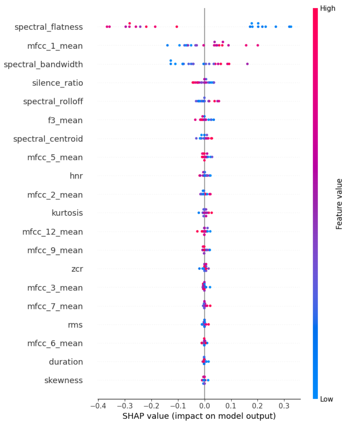
Figura 3.4: Explicación global con SHAP
