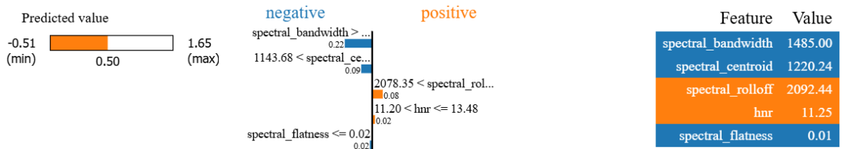
Figura 15: Explicación local espectrales Lime.
