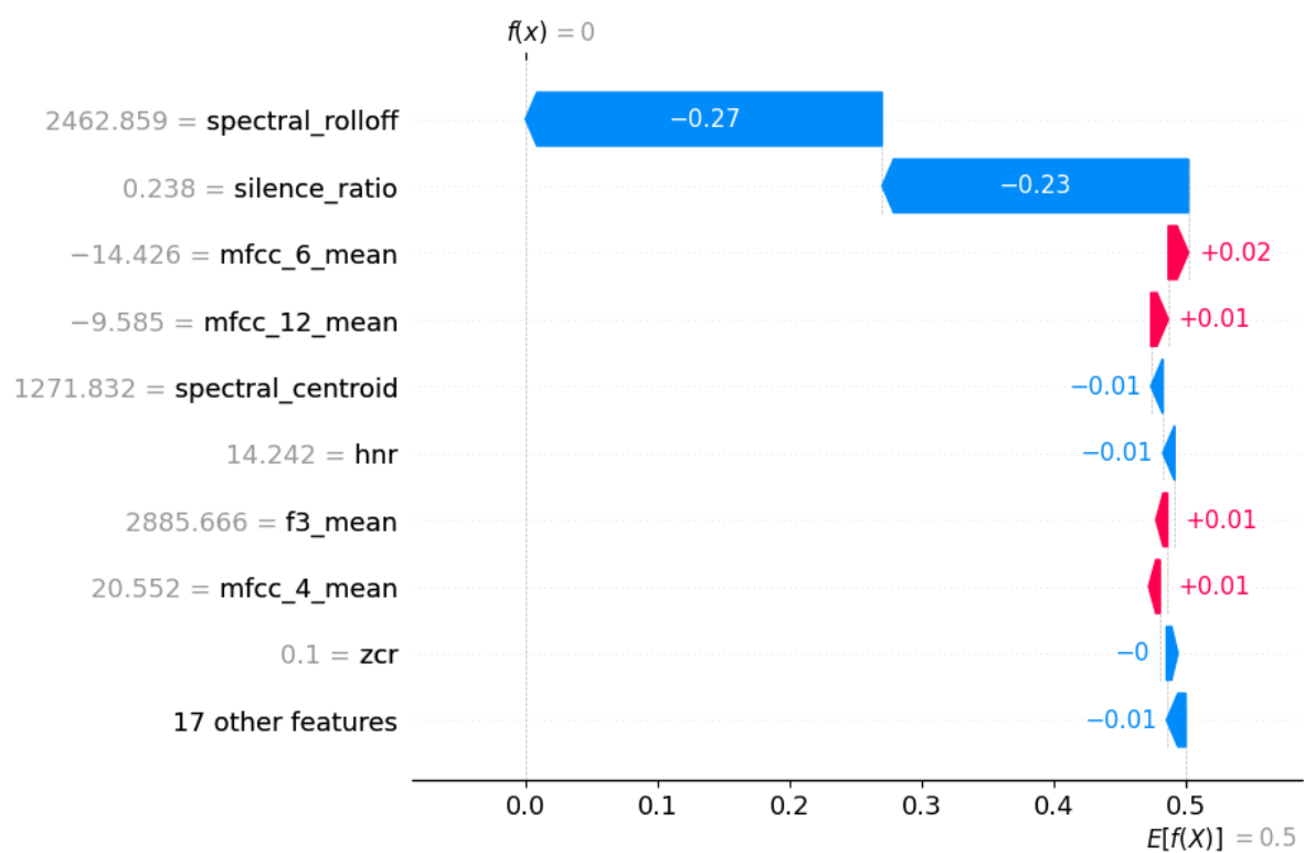
Figura 3.7: Explicación local con SHAP tras quitar spectral flatness, mfcc 1 y spectral bandwidth
