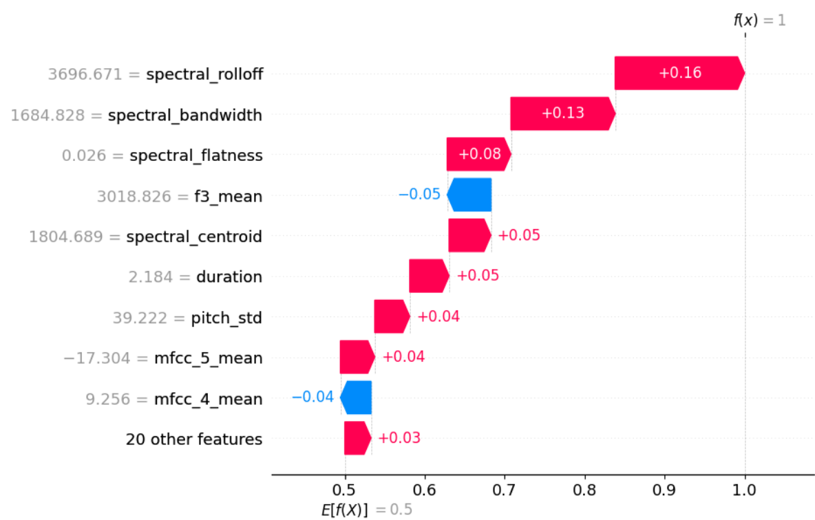
Figura 3.19: Explicación local con SHAP
