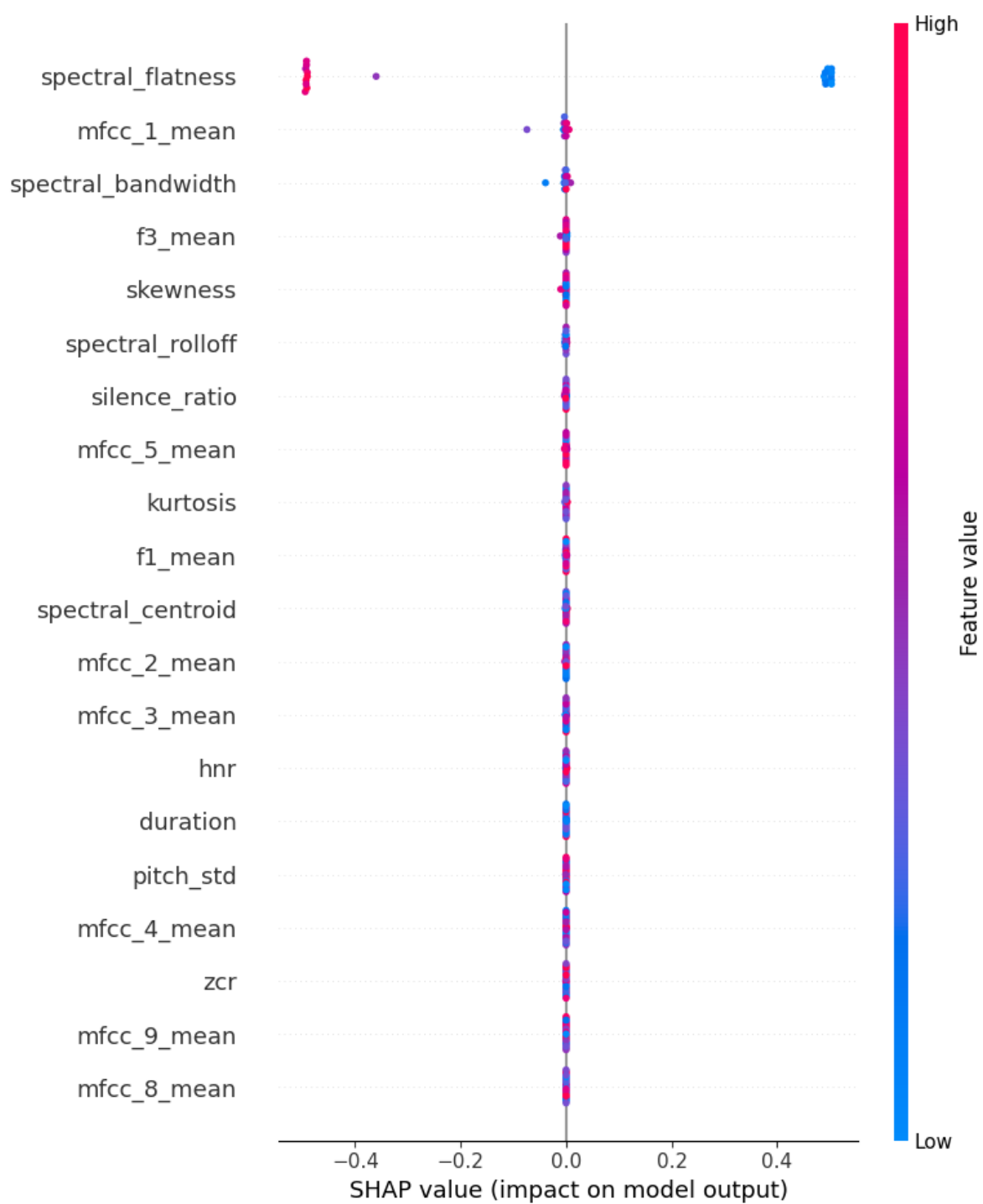
Figura 3.12: Explicación global con SHAP
