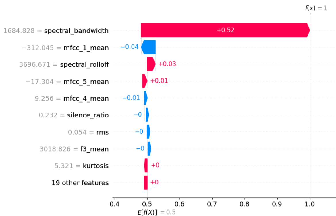
Figura 3.14: Explicación local con SHAP tras quitar spectral flatness
