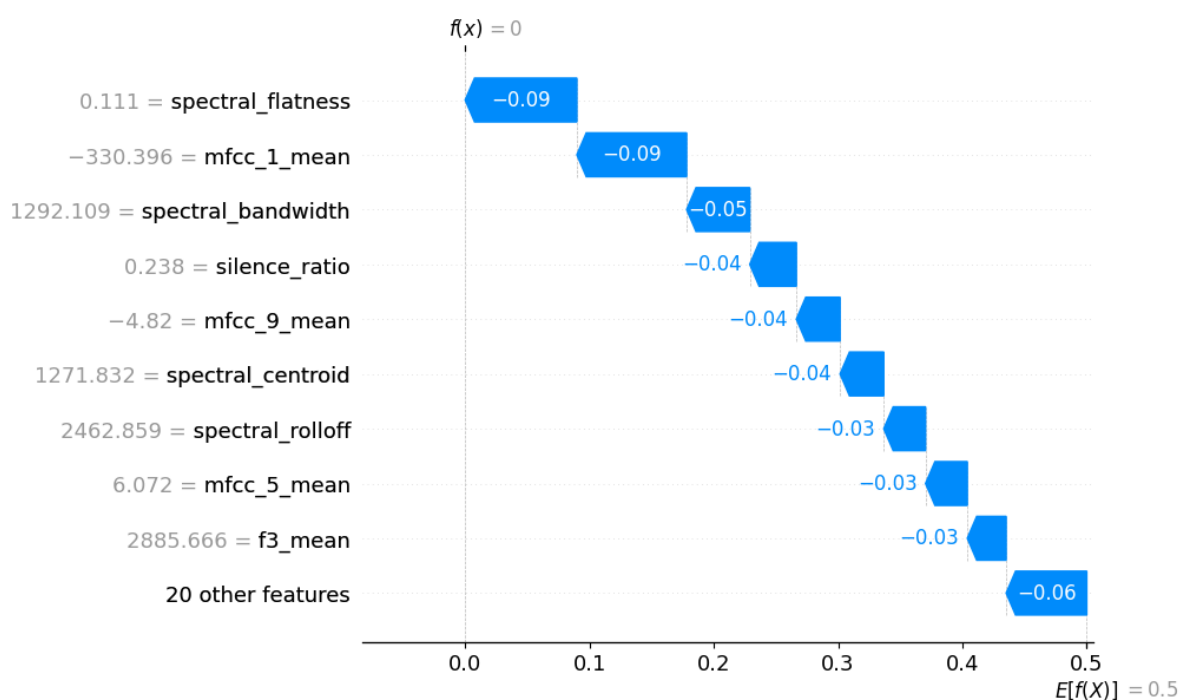
Figura 3.18: Explicación local con SHAP
