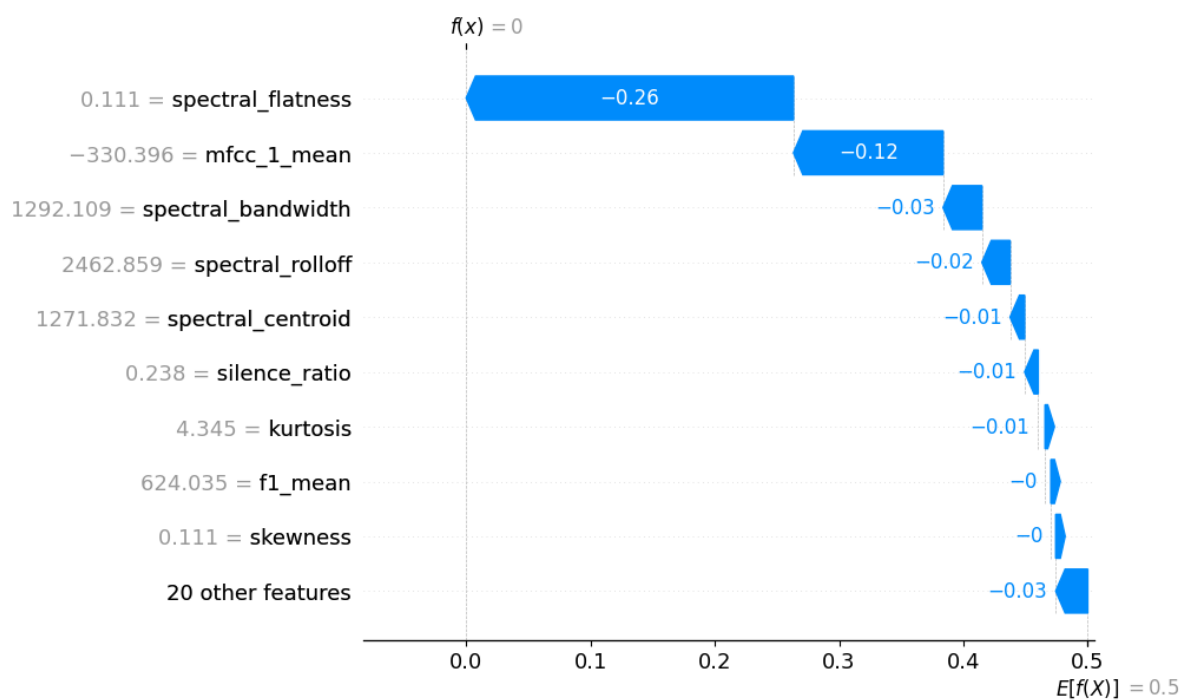
Figura 3.2: Explicación local con SHAP
