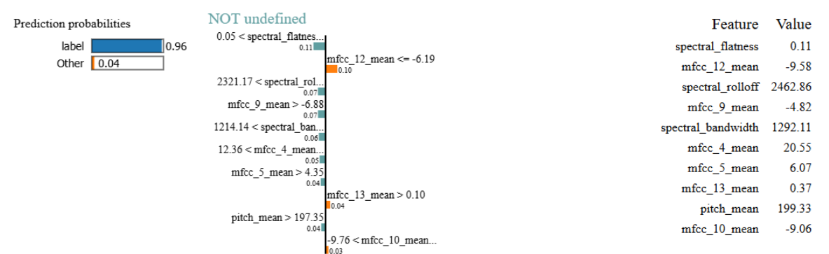
Figura 3.25: Explicación local con LIME
