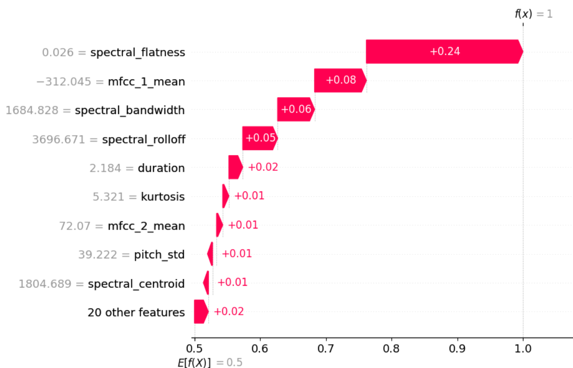
Figura 3.3: Explicación local con SHAP
