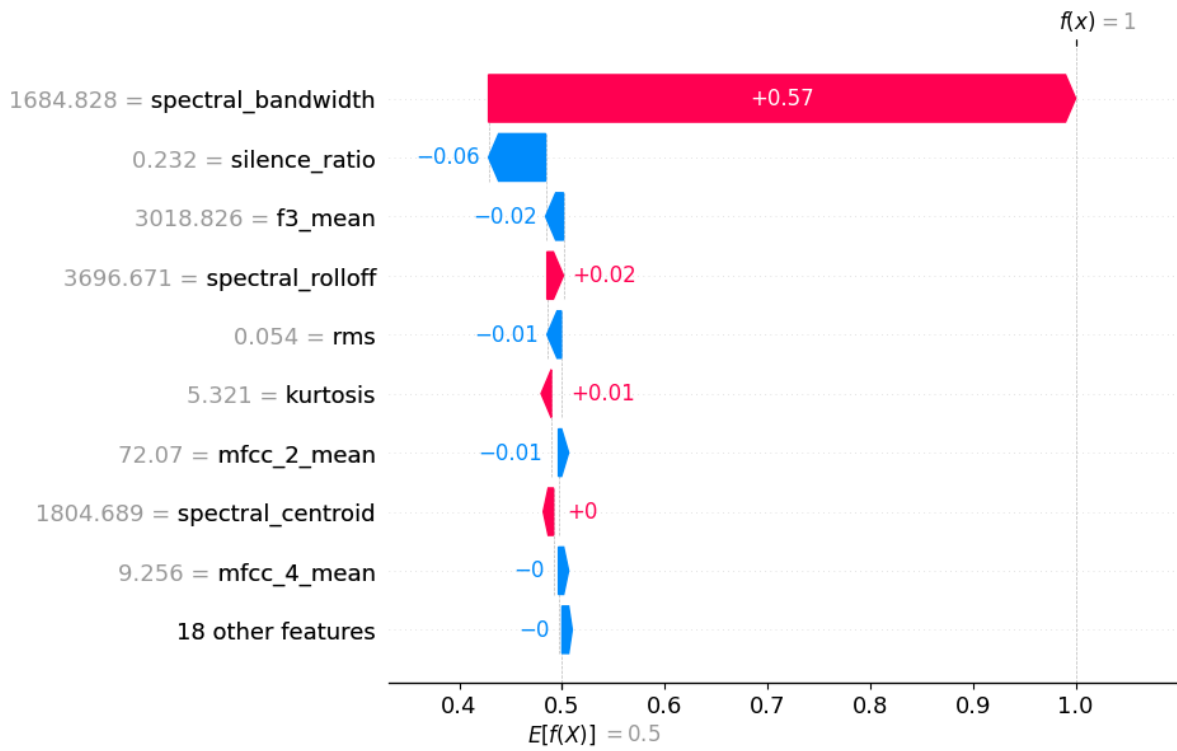
Figura 3.16: Explicación local con SHAP tras quitar spectral flatness y mfcc 1
