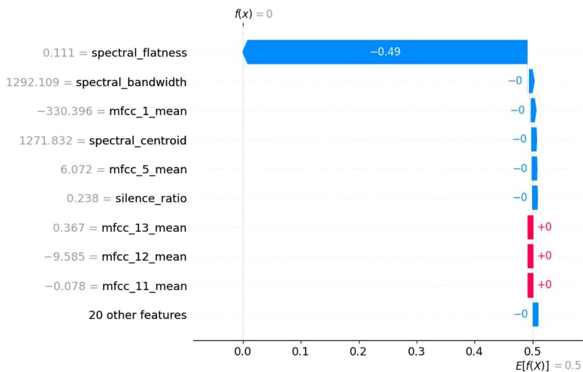
Figura 3.10: Explicación local con SHAP
