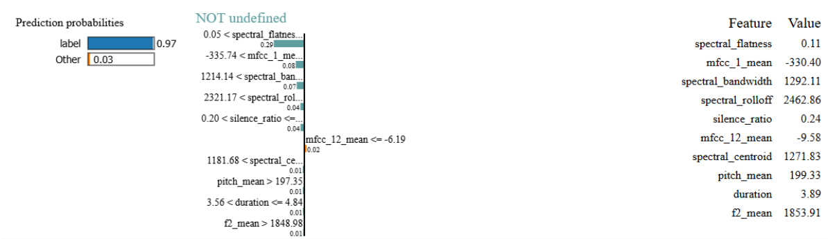
Figura 3.9: Explicación local con LIME
