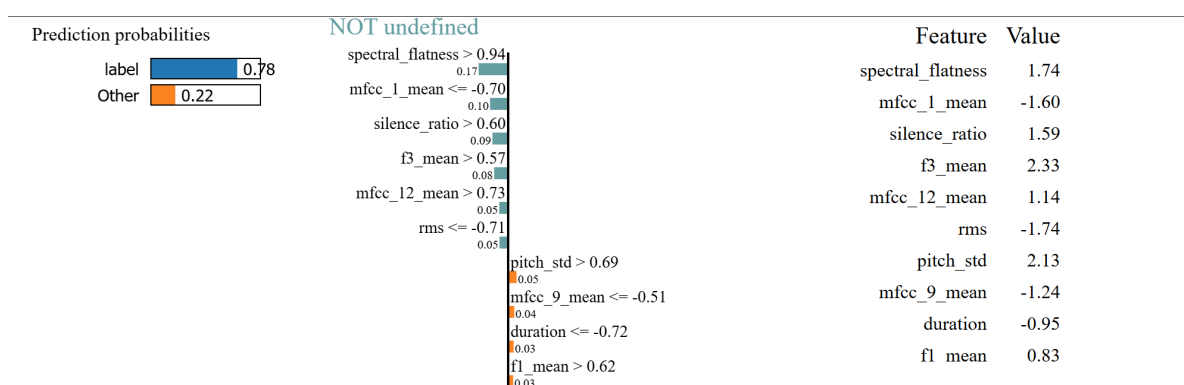
Figura 3.4: Explicación local generada por LIME para el modelo KNN.
