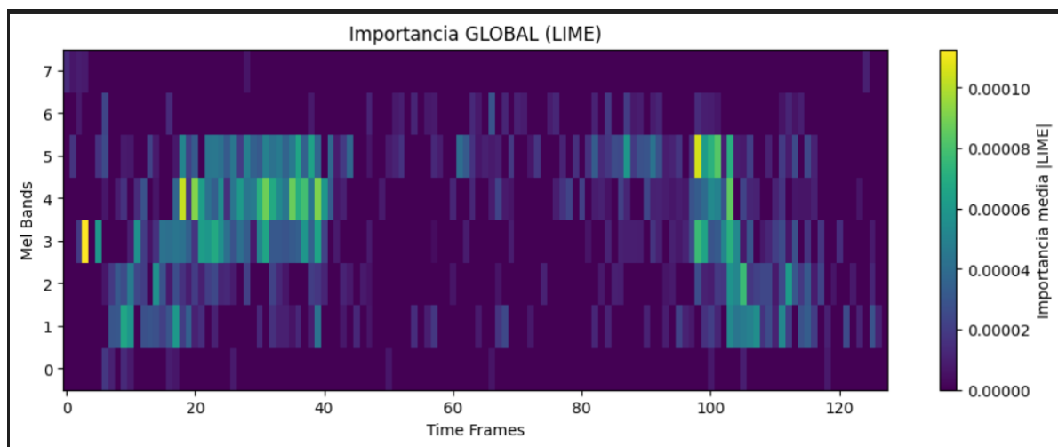
Figura 3.27: Lime general de los espectrogramas
