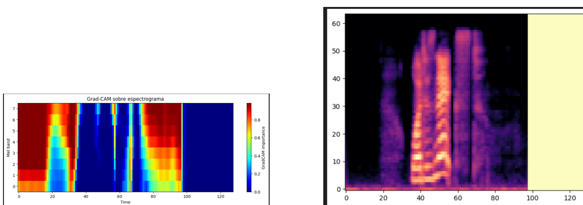
(a) Grad Cam de un audio.
