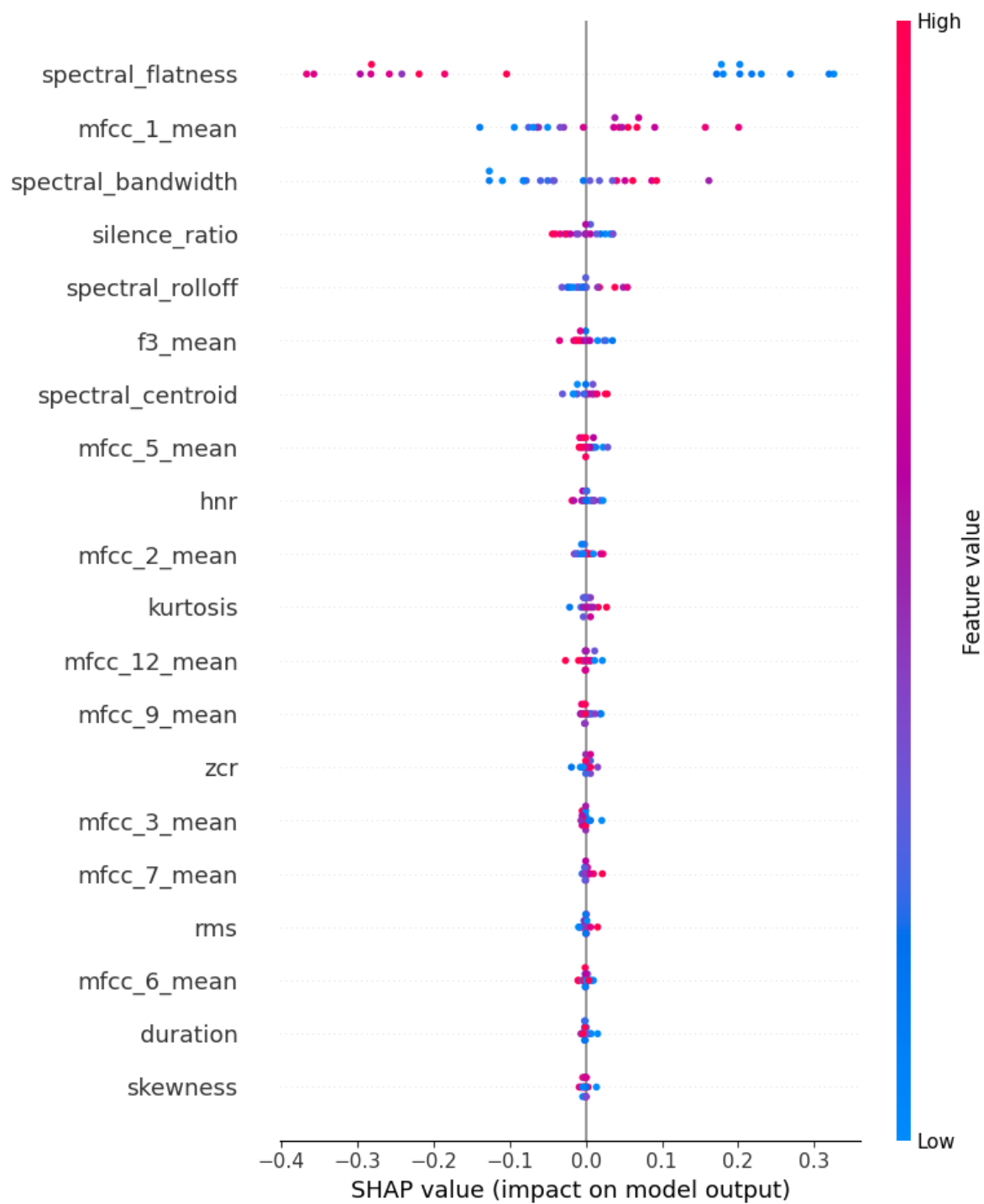
Figura 16: Explicación global de Random Forest con SHAP
