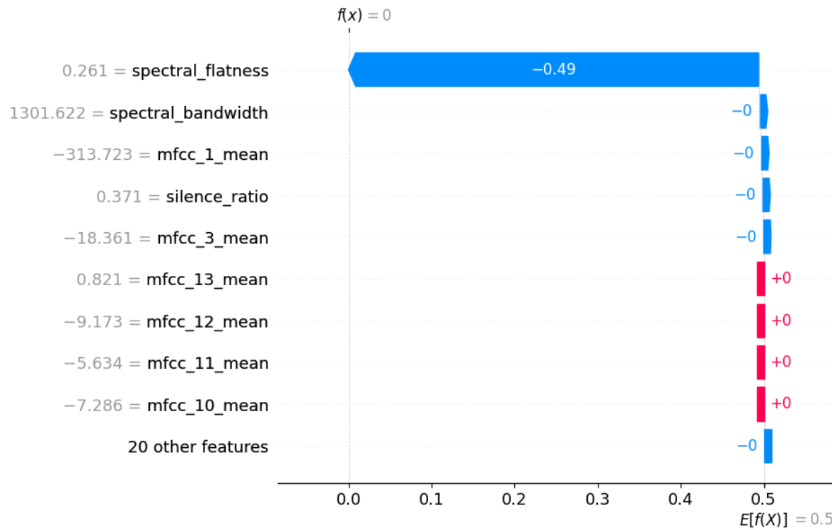
Figura 44: Explicación local de LGBM con SHAP para audios nuevos en español
