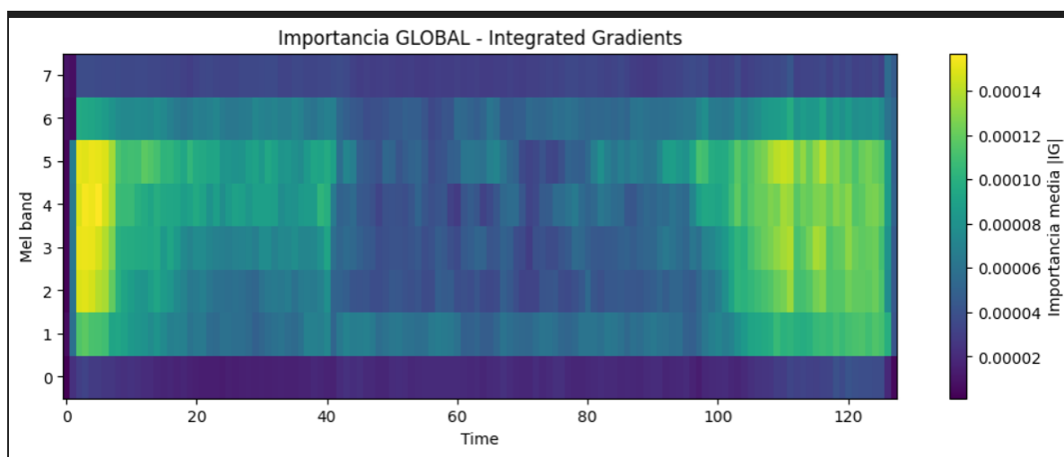
Figura 3.29: Integrated Gradients general de los espectrogramas
