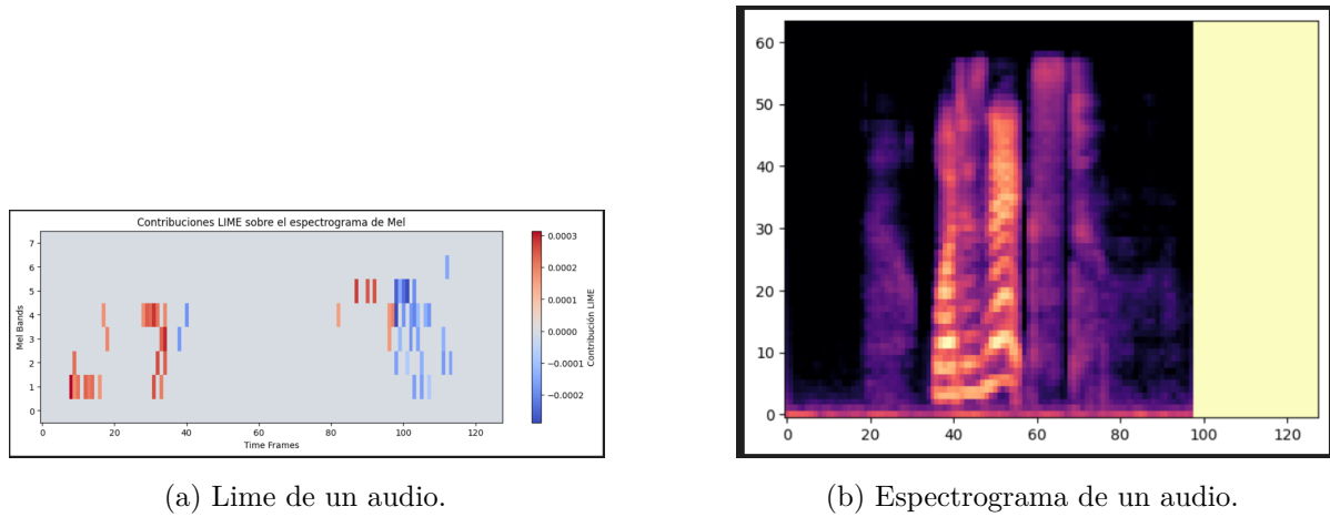
Figura 3.26: Lime local sobre los espectrogramas con Wav2Vec2
