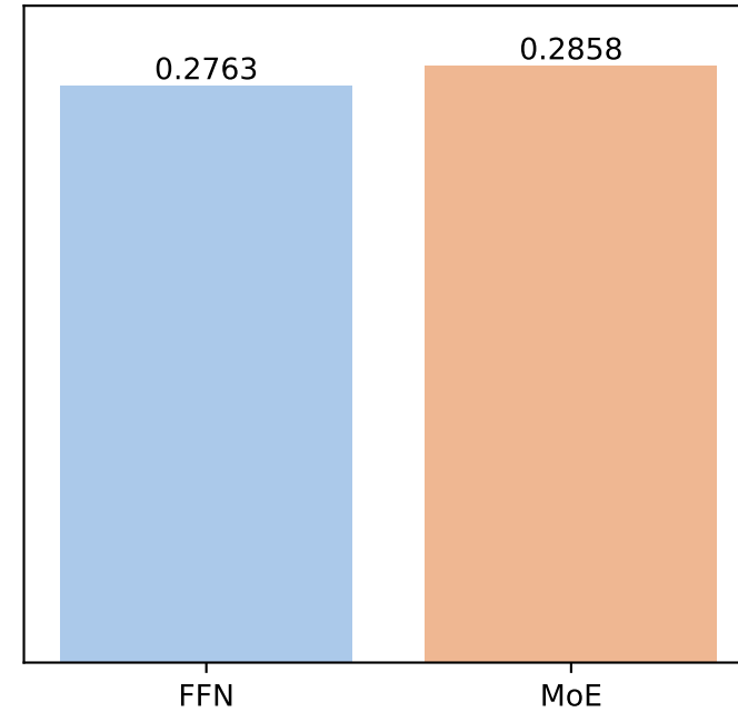
Precision
