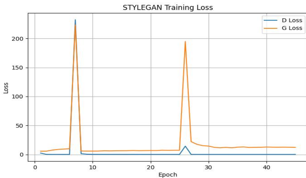
图 7: StyleGAN 训练曲线 (明显看出超参数问题导致的崩溃)
