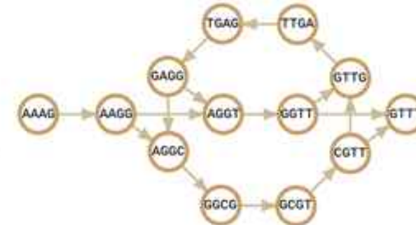
C Hamiltonian de Bruijn graph
