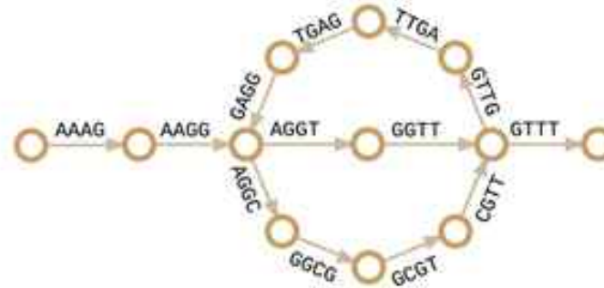
B Eulerian de Bruijn graph
