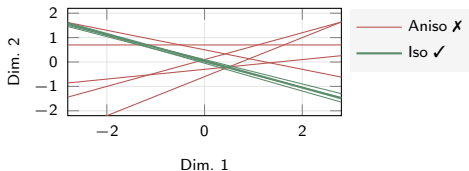
Variance của decision boundary
