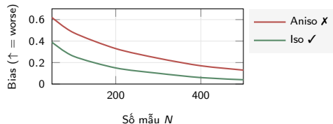
Bias theo số mẫu N
