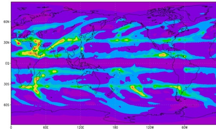
Precipitation 720hr
