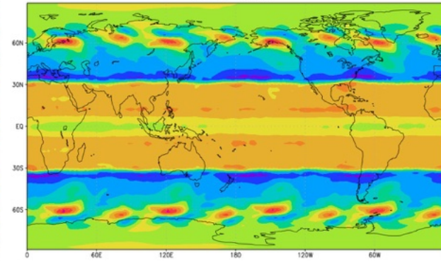
UGRD 120hr
