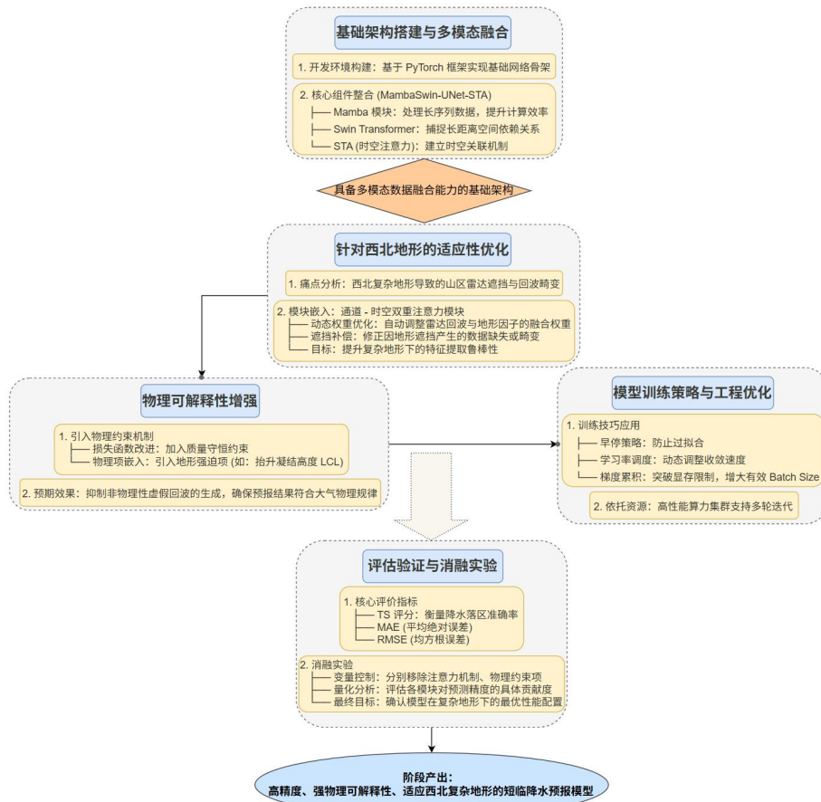
图 11 基于时空注意力机制的短临预报模型设计技术路线图
