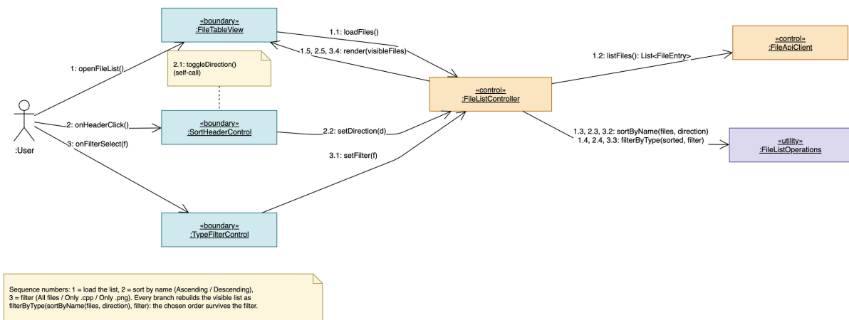
Рисунок 9. Діаграма комунікації: сортування і фільтр
