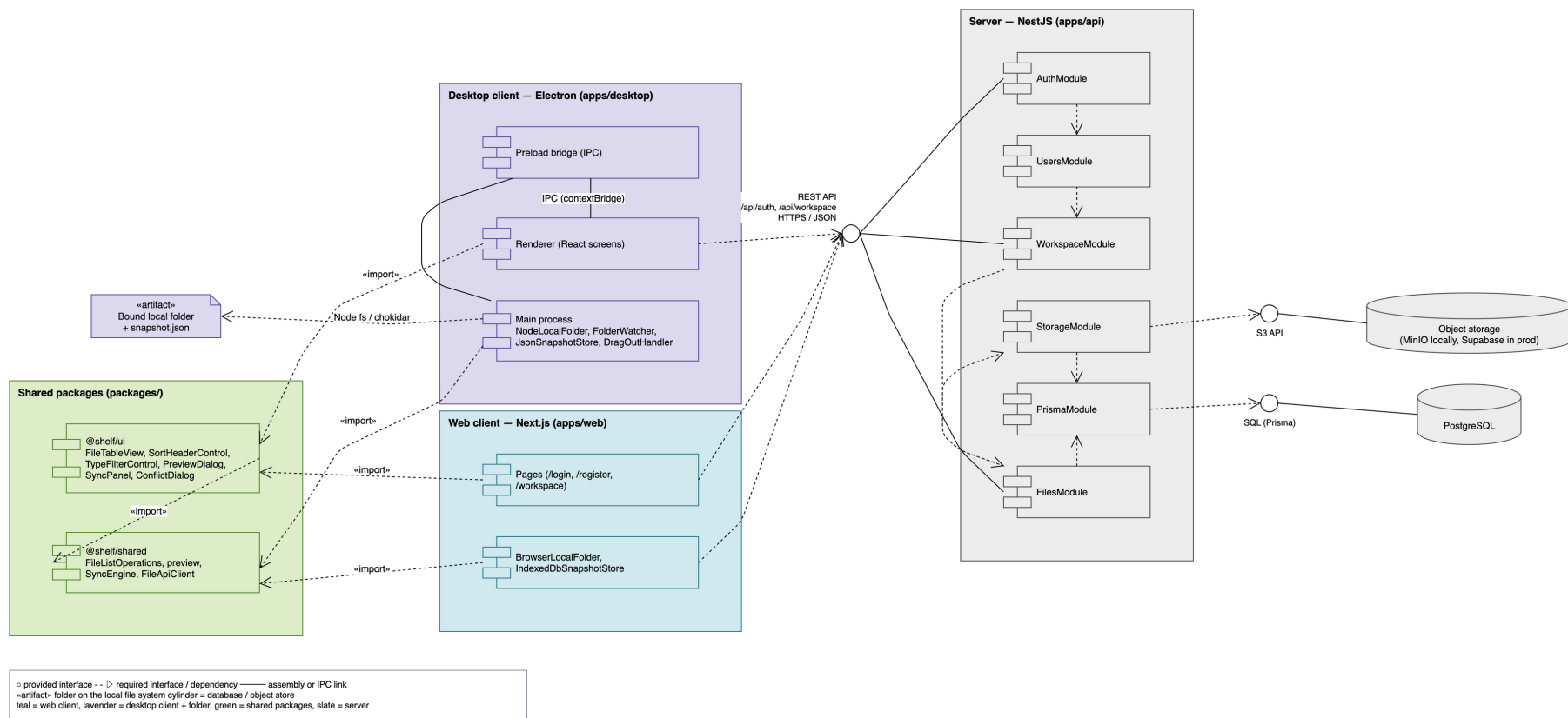
Рисунок 1. Діаграма компонентів
