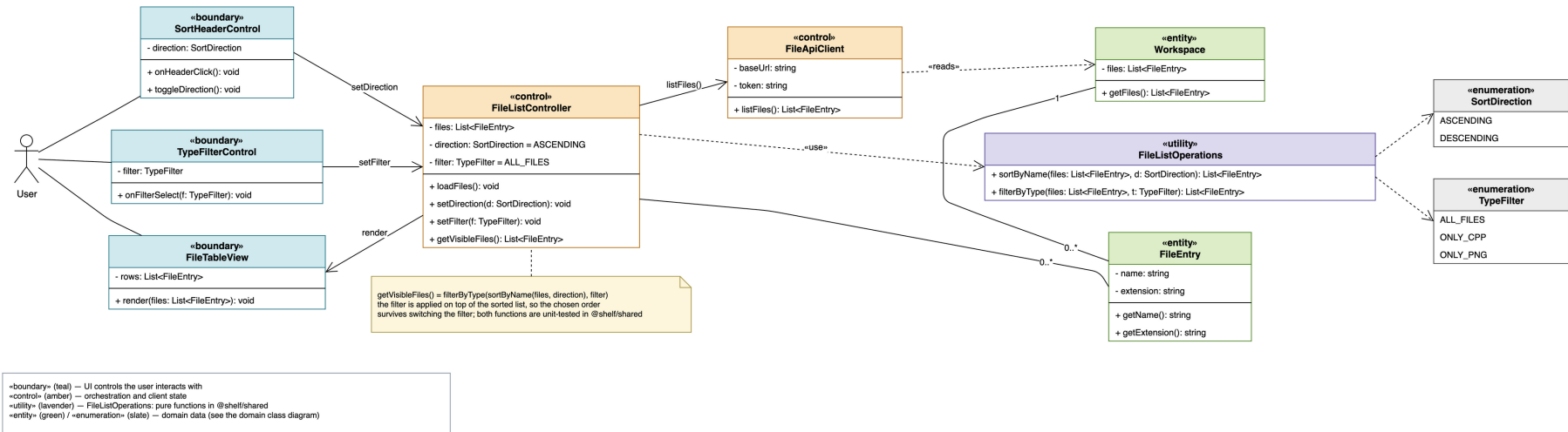
Рисунок 5. Діаграма класів VOPC: сортування і фільтр
