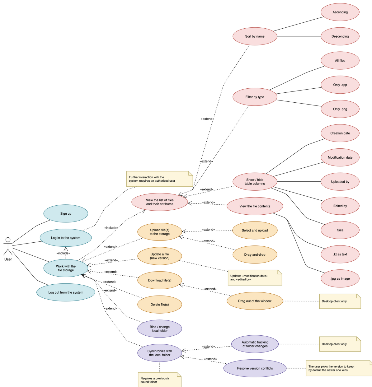
Рисунок 3. Діаграма прецедентів
