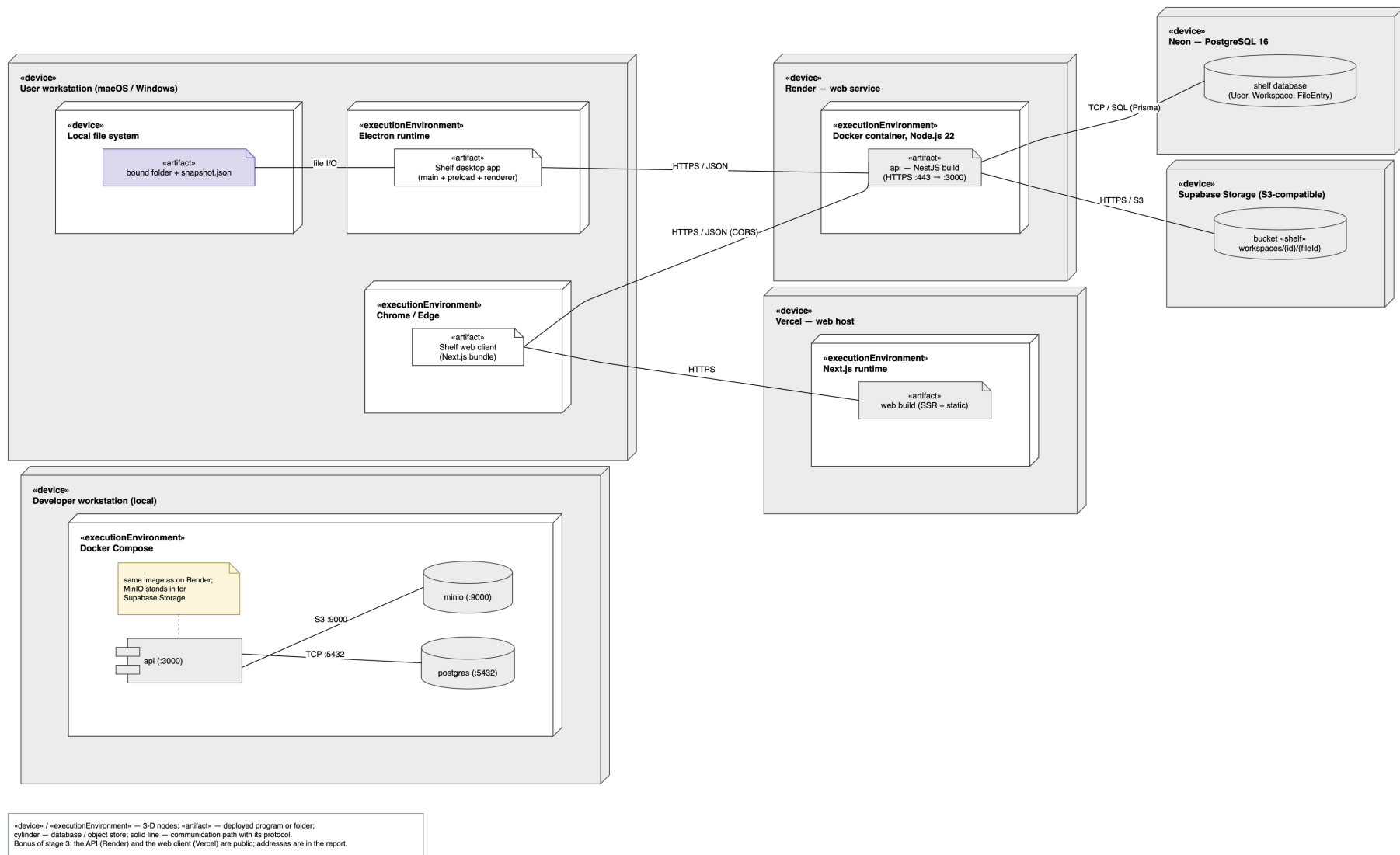
Рисунок 2. Діаграма розгортання
