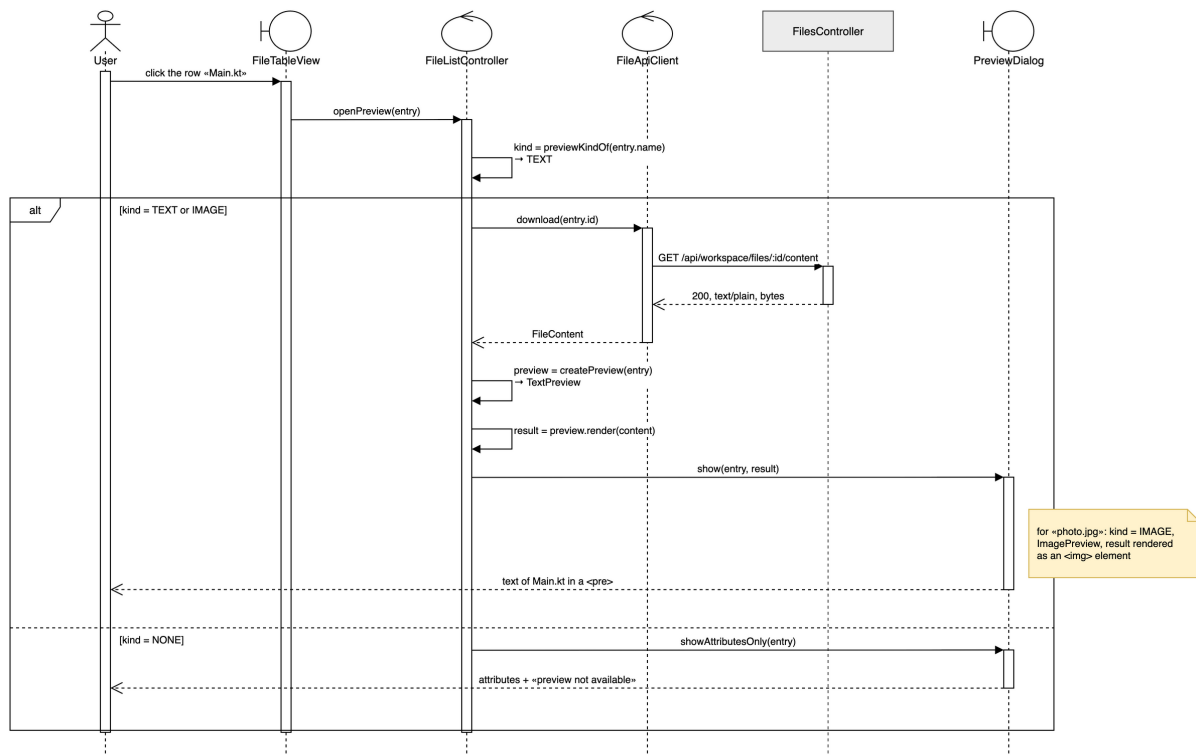
Рисунок 6. Діаграма послідовності: перегляд вмісту файлу
