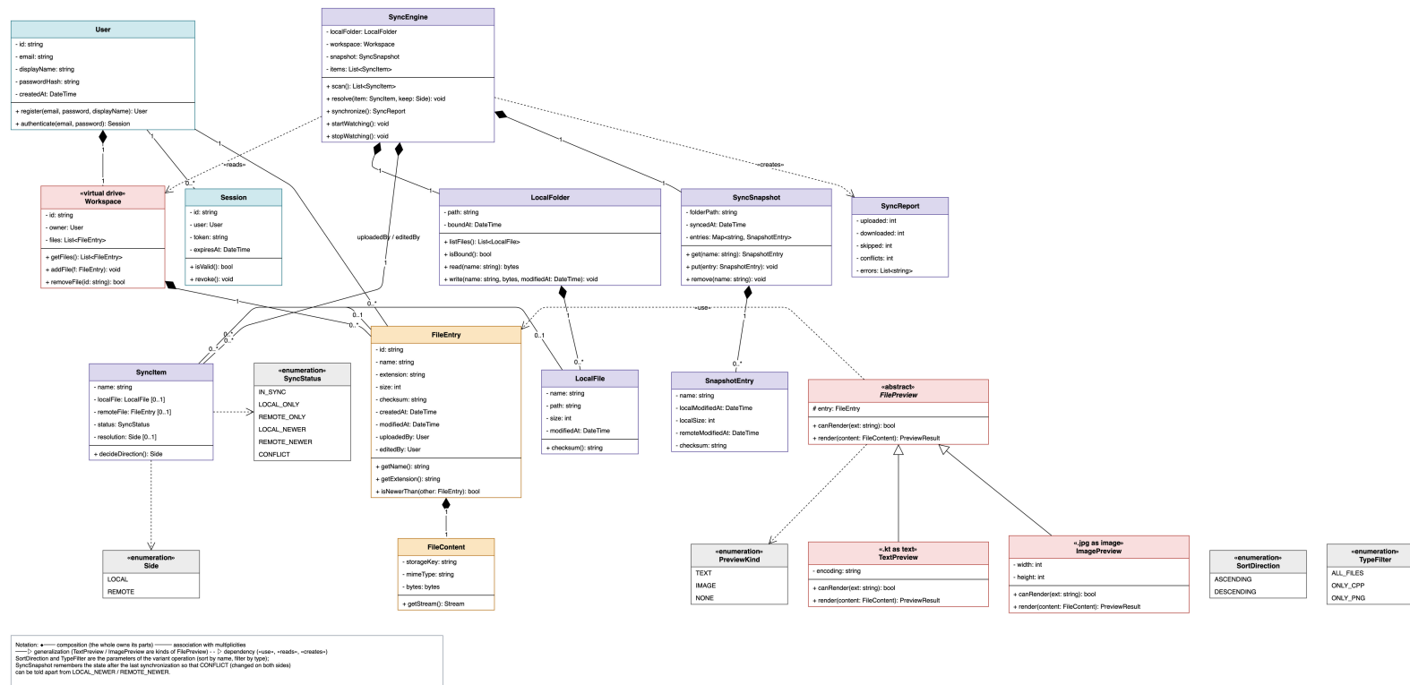
Рисунок 2. Діаграма класів: доменна модель
