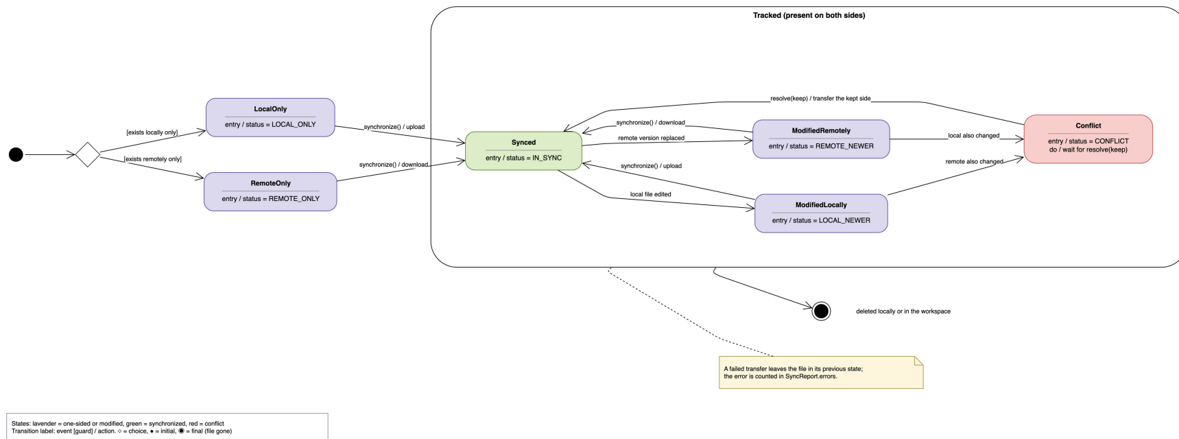
Рисунок 8. Діаграма станів файлу
