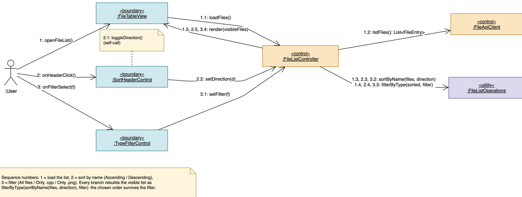
Рисунок 7. Діаграма комунікації: сортування і фільтр
