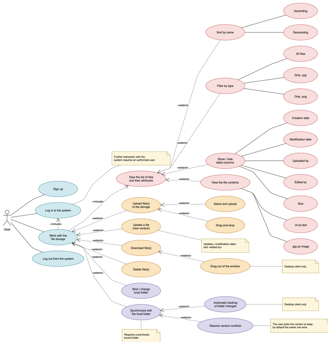
Рисунок 1. Діаграма прецедентів
