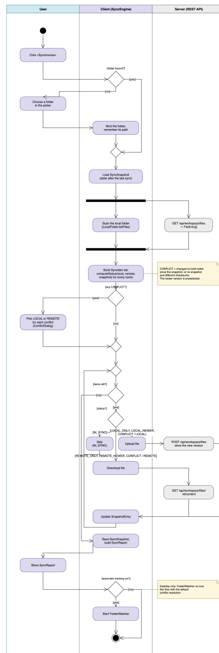
Рисунок 4. Діаграма активності: синхронізація
