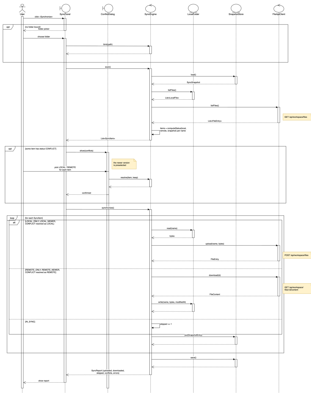
Рисунок 5. Діаграма послідовності: синхронізація
