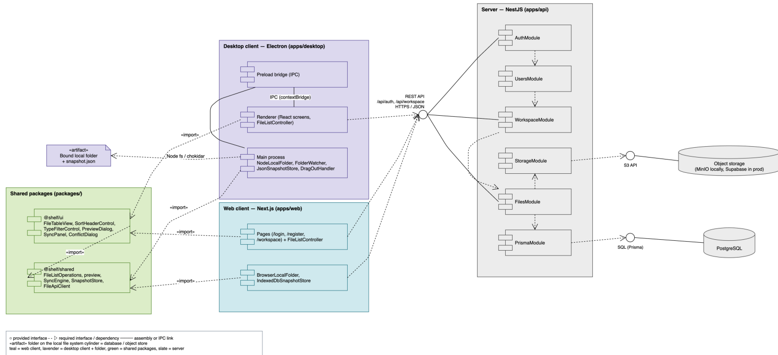
Рисунок 9. Діаграма компонентів
