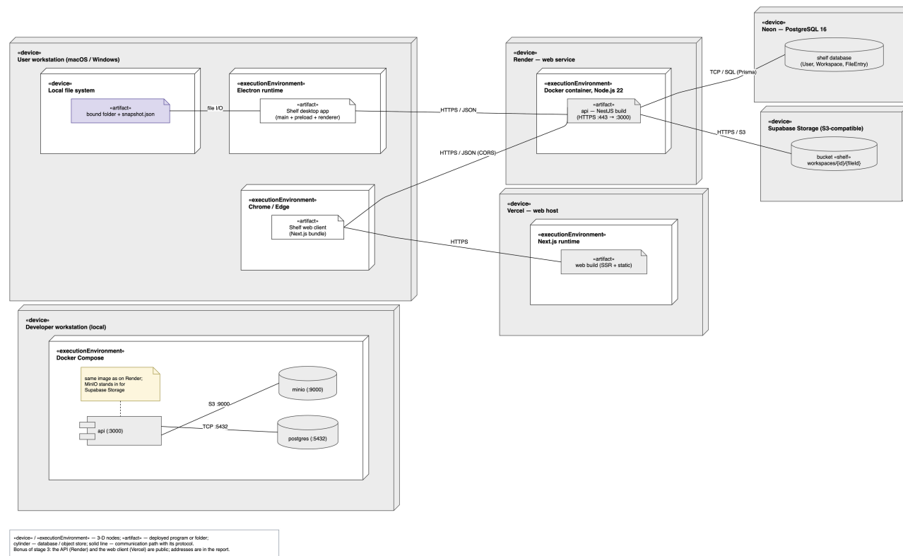
Рисунок 2. Діаграма розгортання
