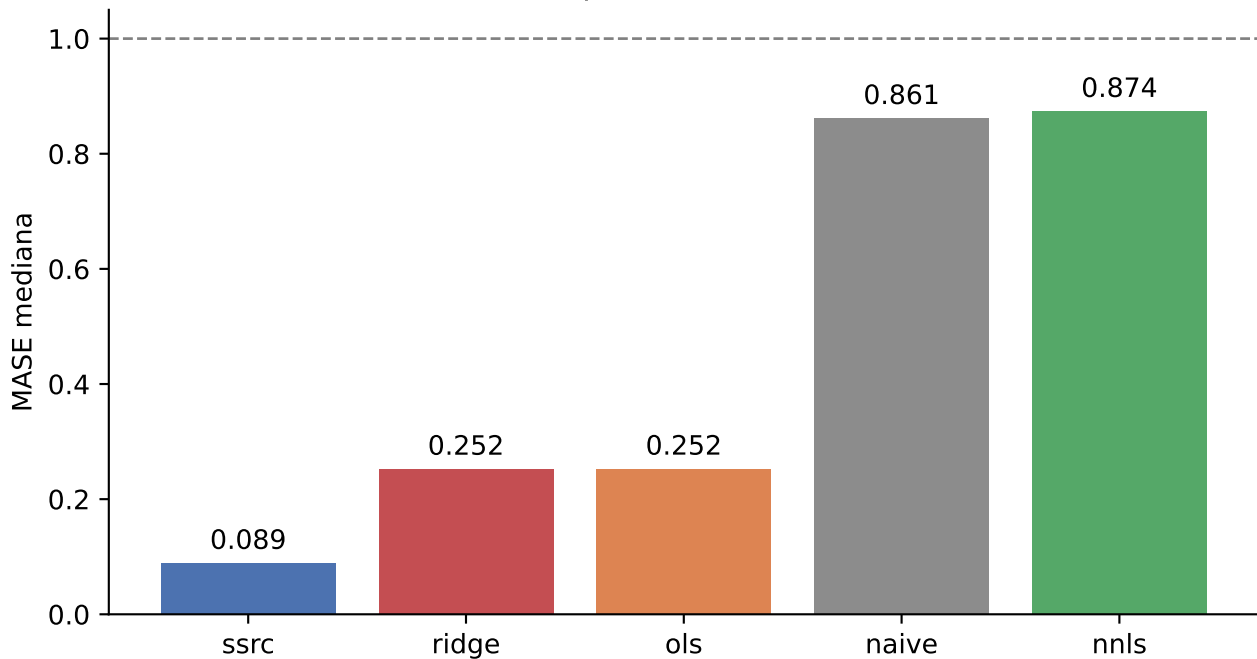
Lorenz63: comparación causal de lectores
