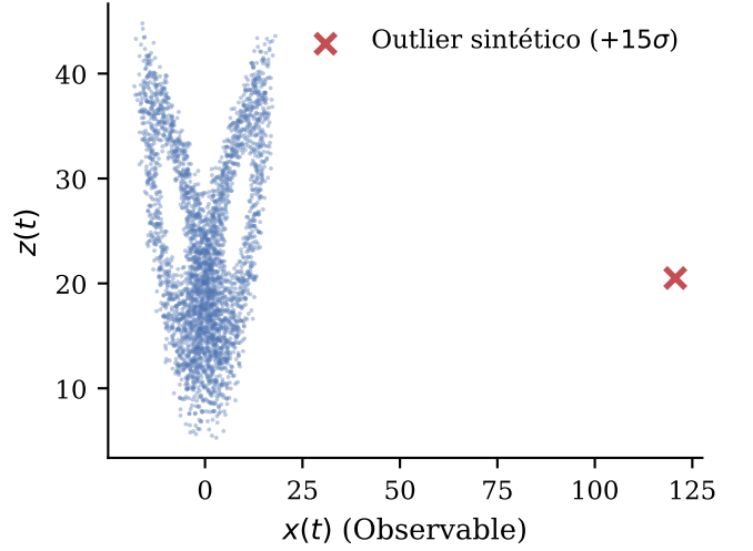
Lorenz63: Atractor y Shock Fuera del Manifold
