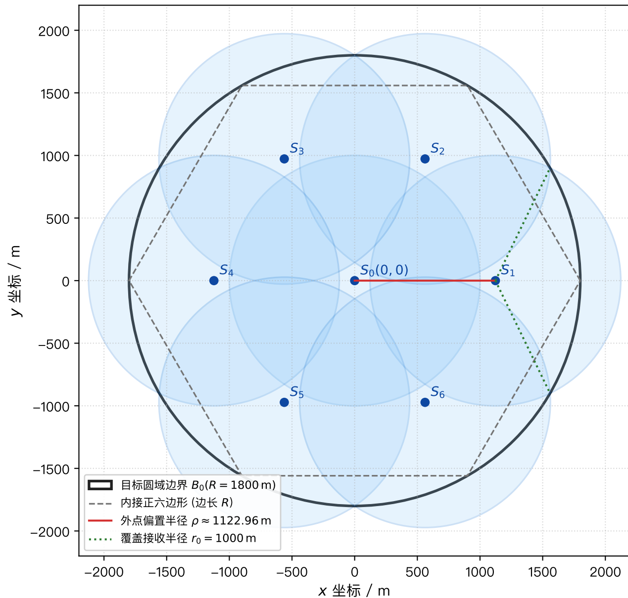
(a) 七点覆盖几何布局与最小接收半径保证
