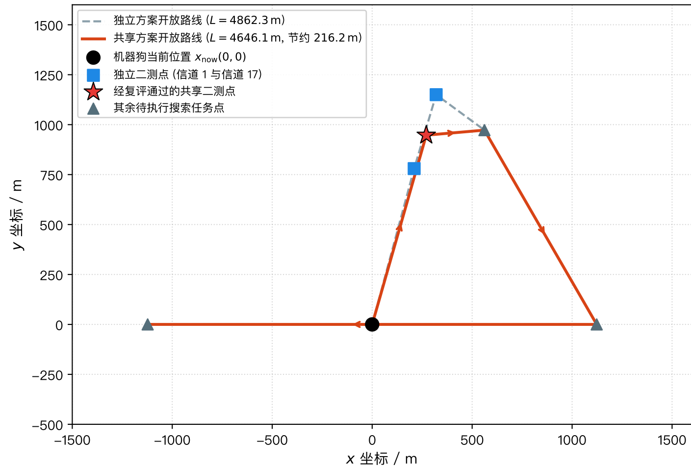
(b) 同一任务快照下共享二测与开放 TSP 路线对比
