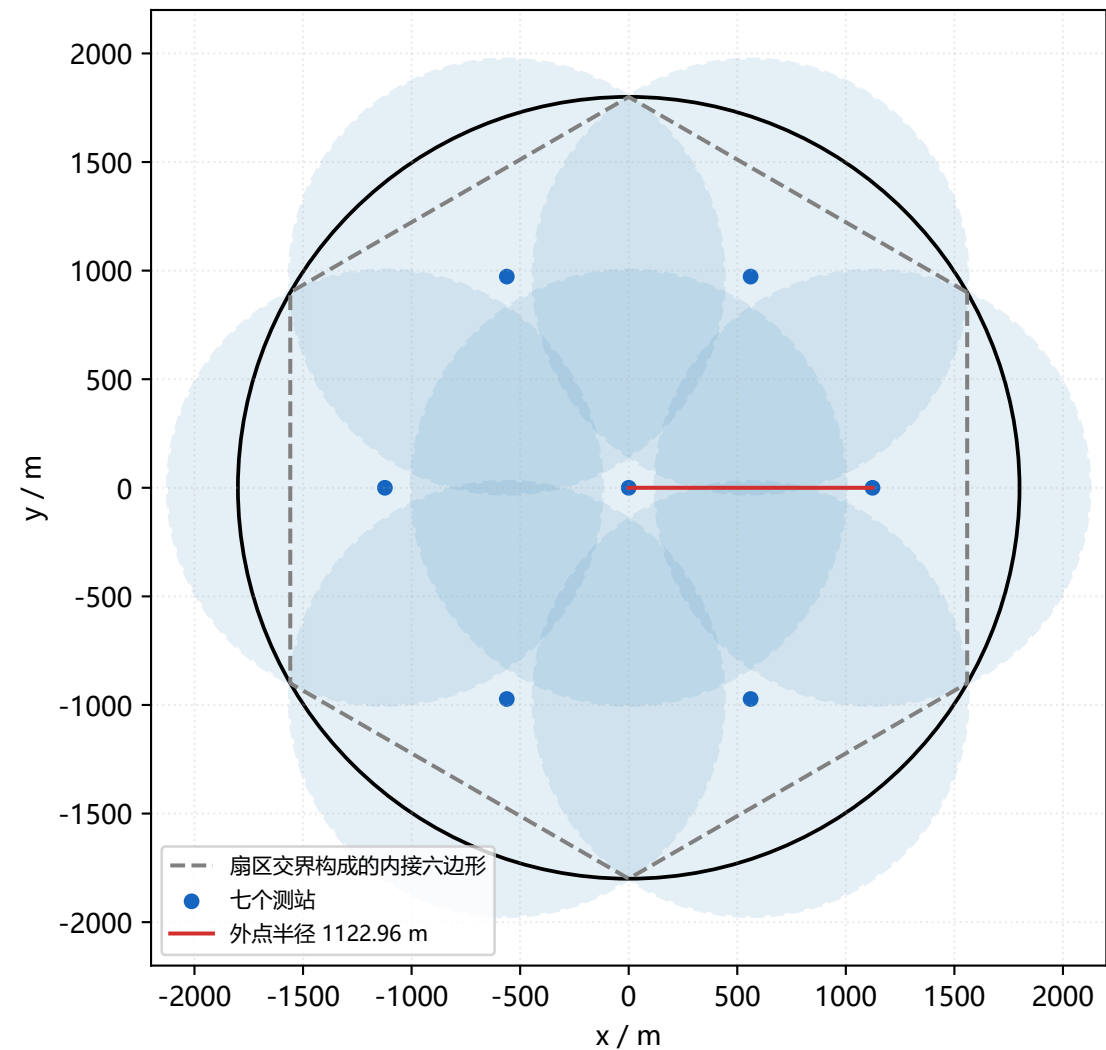
(a) 七点覆盖: 接收半径 1000 m
