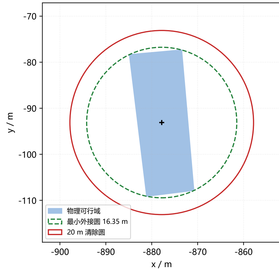
(a) 2 次测向 · 已满足几何覆盖
