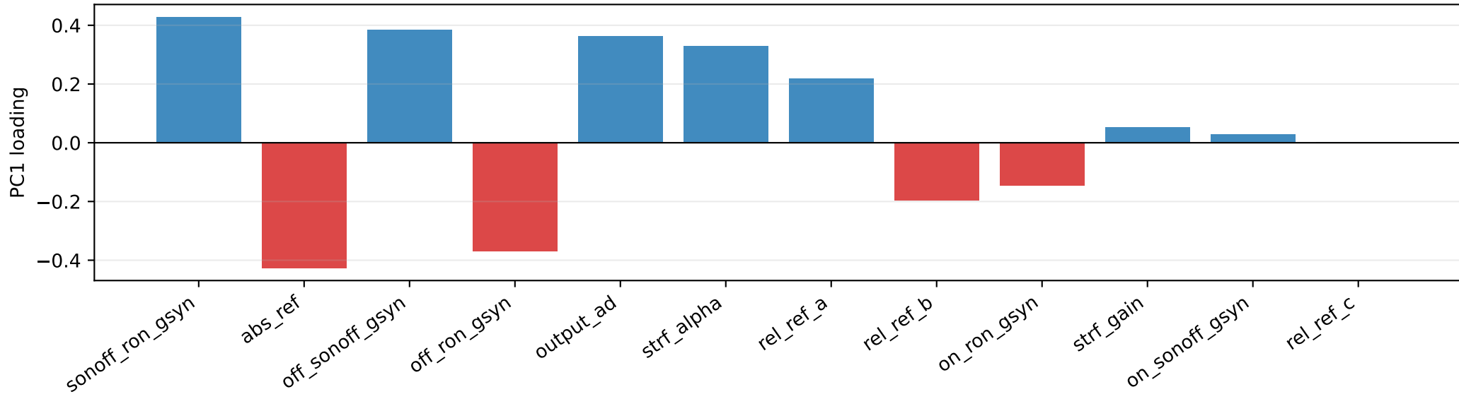
PC1 parameter loadings, standardized parameter units
