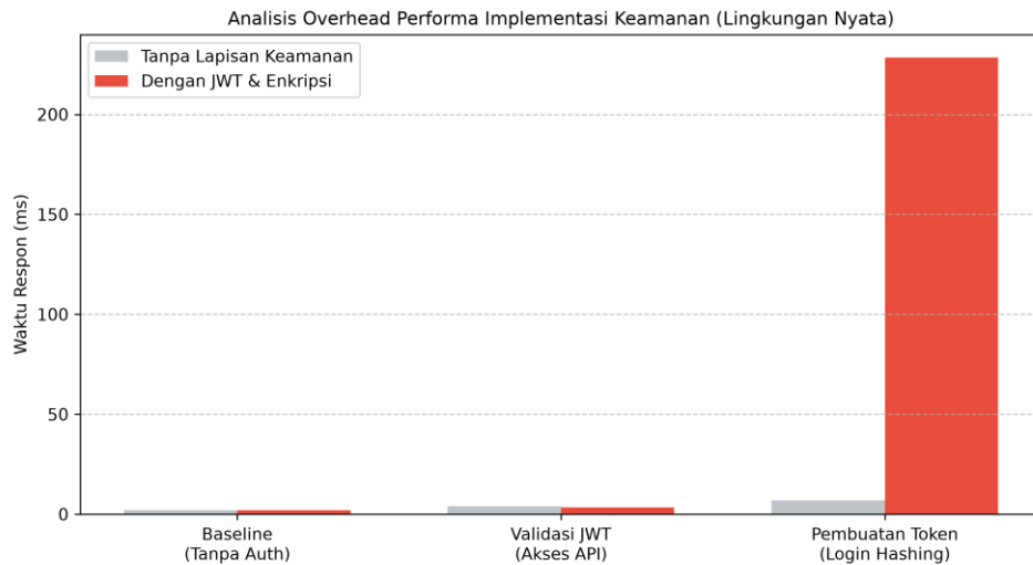
Gambar 1. Analisis Dampak Latensi dari Pemasangan Mekanisme Keamanan
