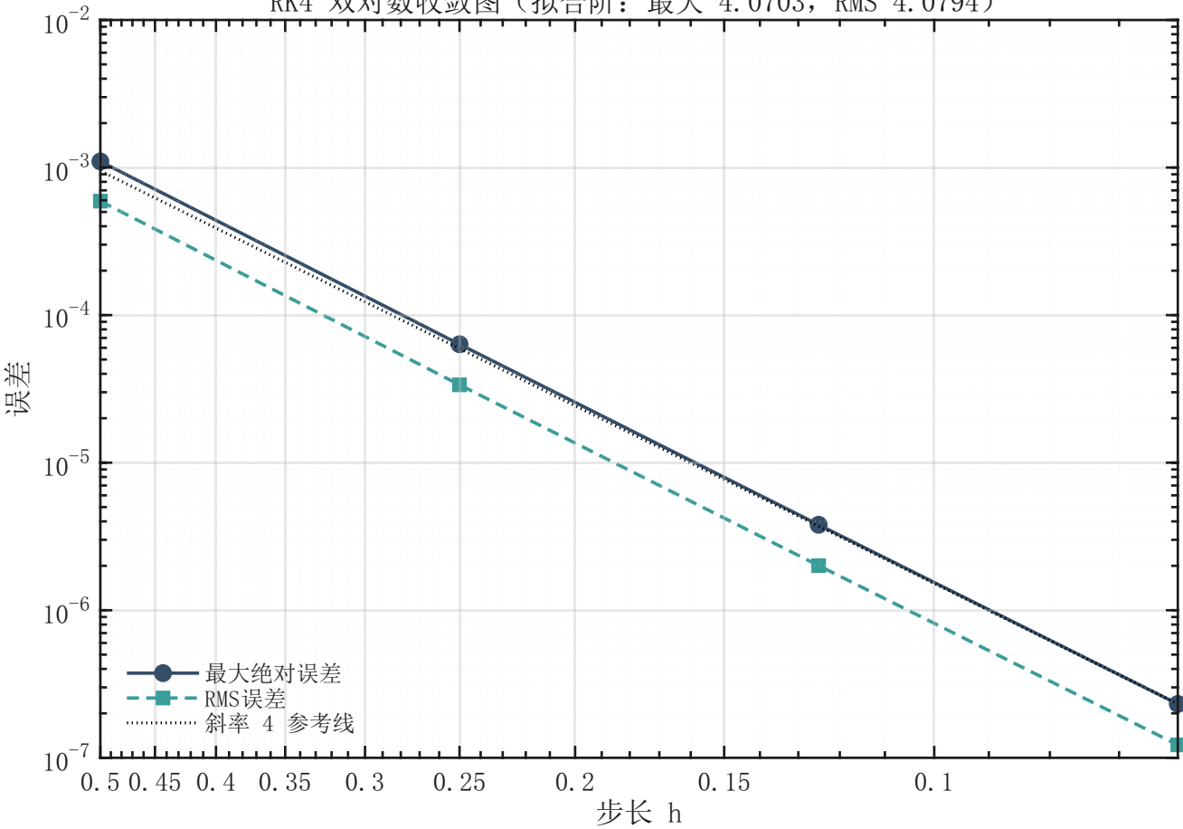
RK4 双对数收敛图 (拟合阶: 最大 4.0703, RMS 4.0794)
