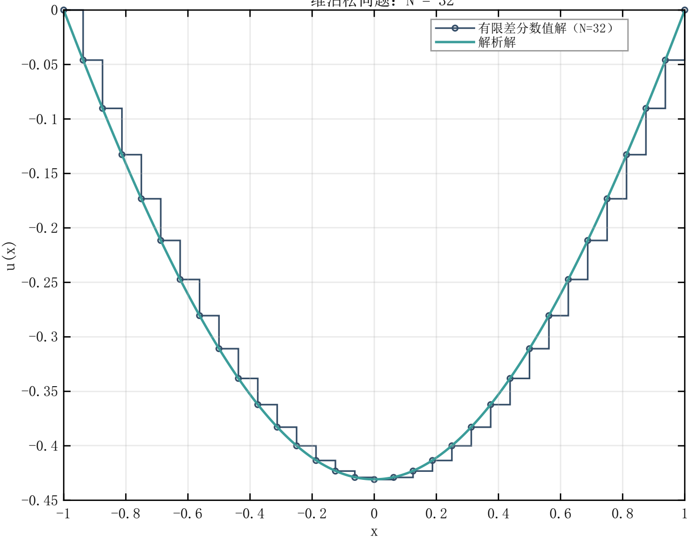
一维泊松问题：N = 32
