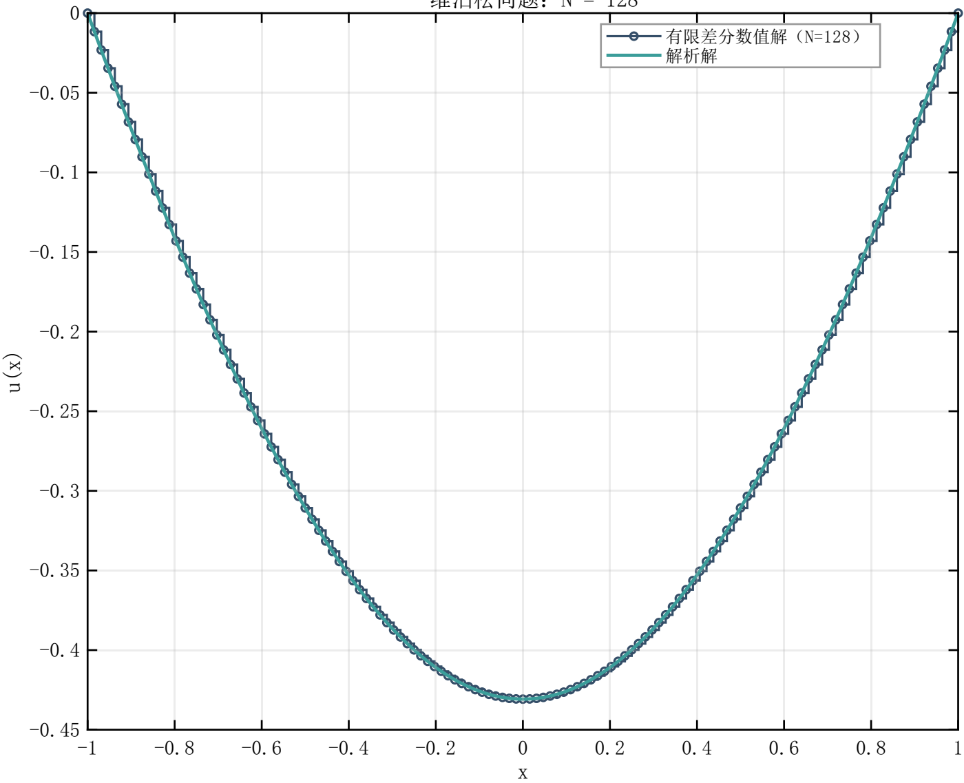
一维泊松问题: N = 128
