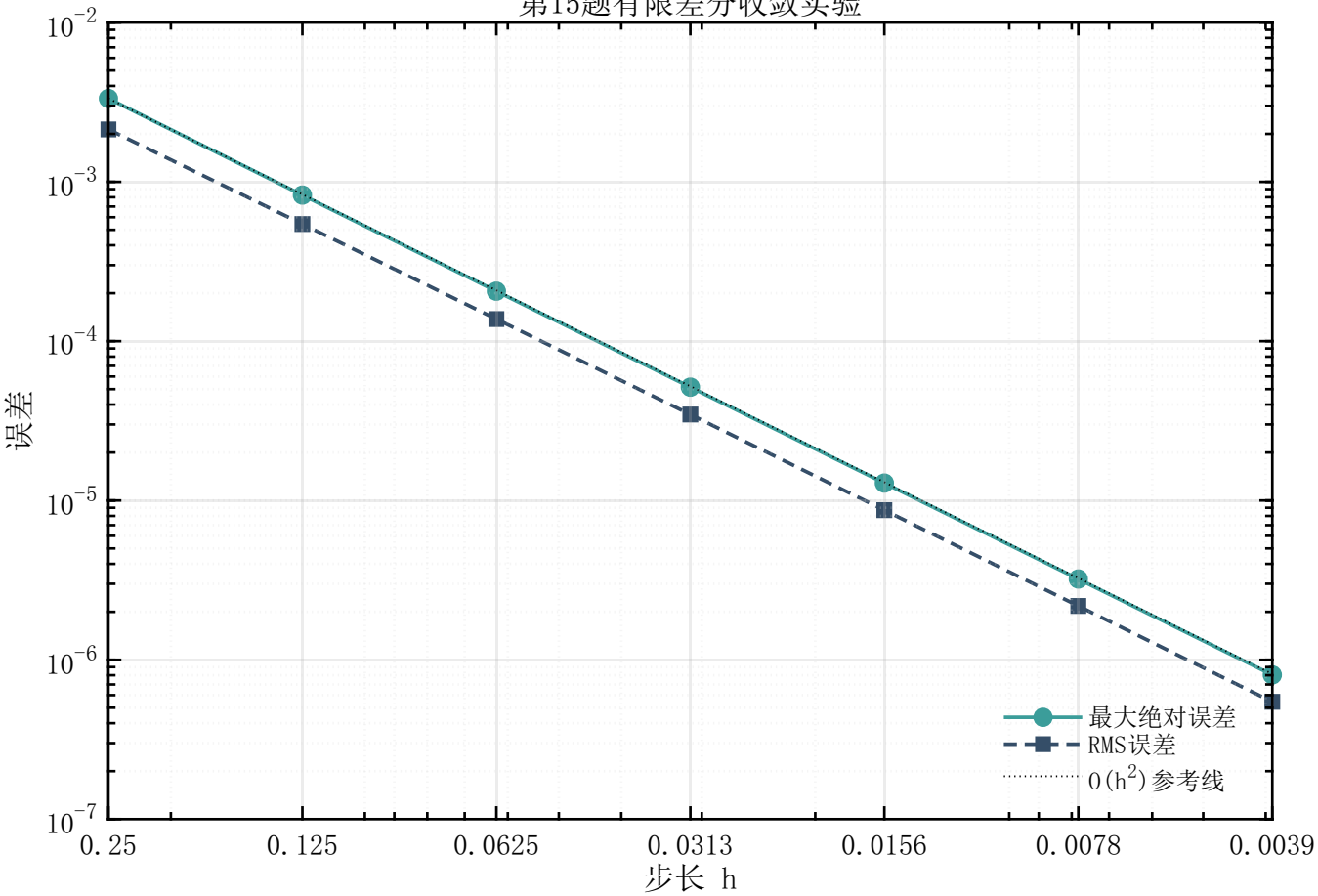
第15题有限差分收敛实验
