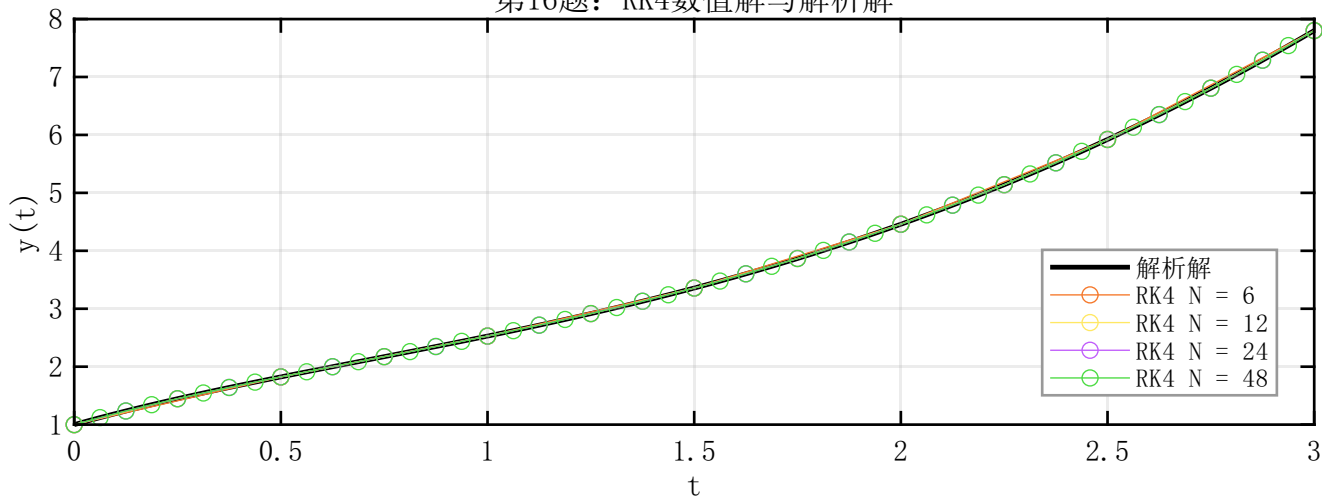
第16题：RK4数值解与解析解
