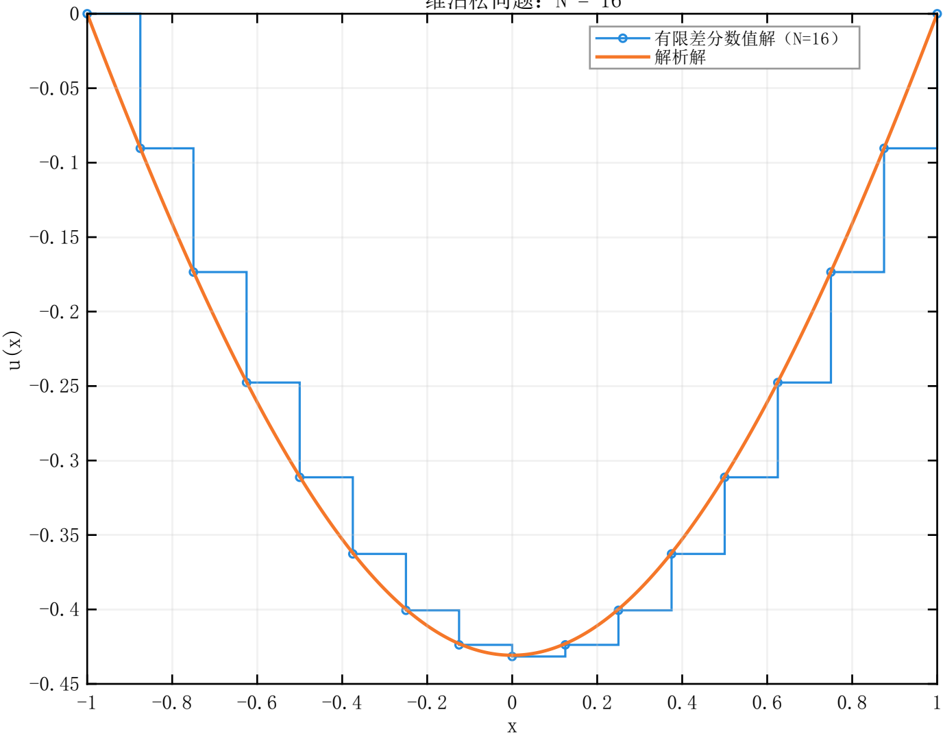
一维泊松问题: N = 16
